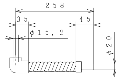
本体側 ドレンホース (本体同梱)
