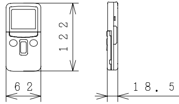
ワイヤレスリモコン
