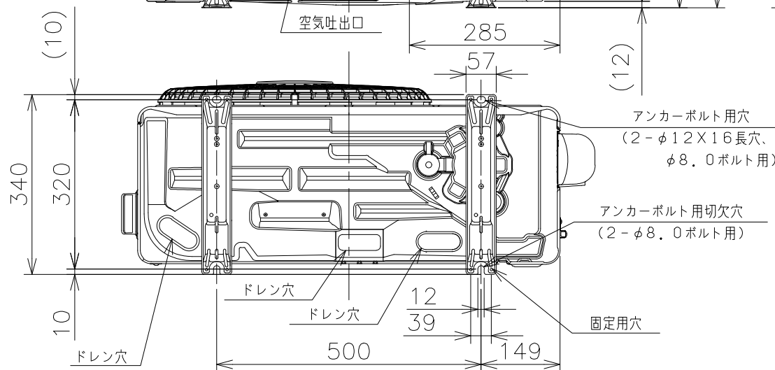
背面図
