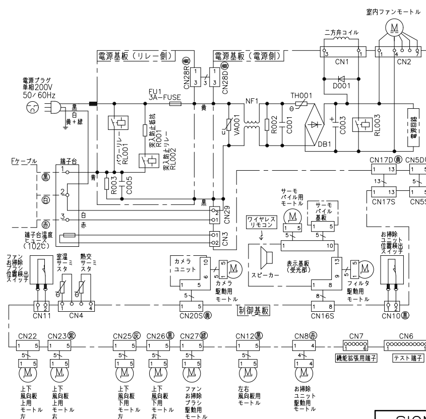
配線図 RAS-VL71K2EE
