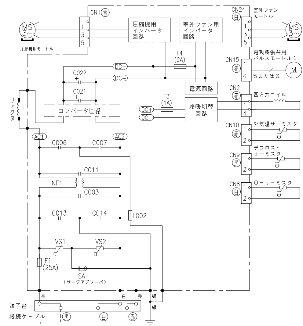
配線図 RAC-VL71K2EE
