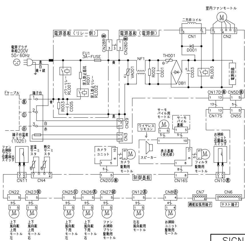
配線図 RAS-VL63K2EE
