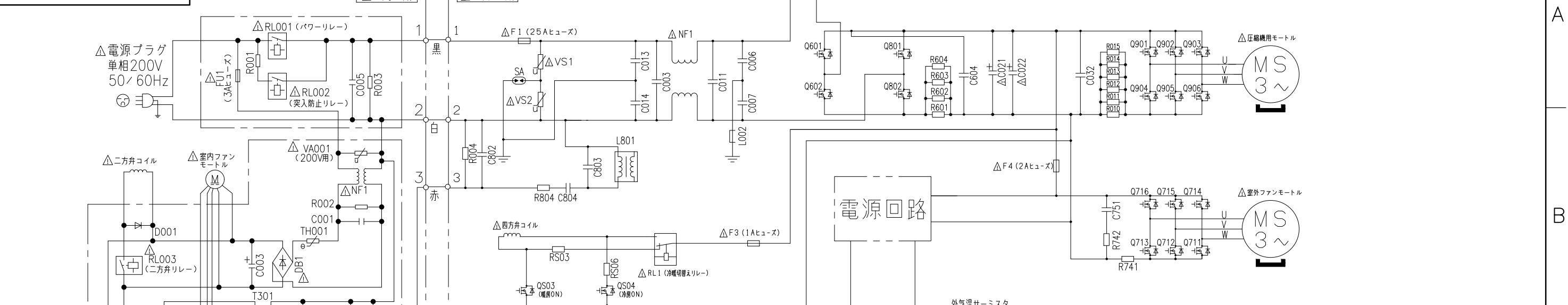
配線図 RAC-VL63K2EE
