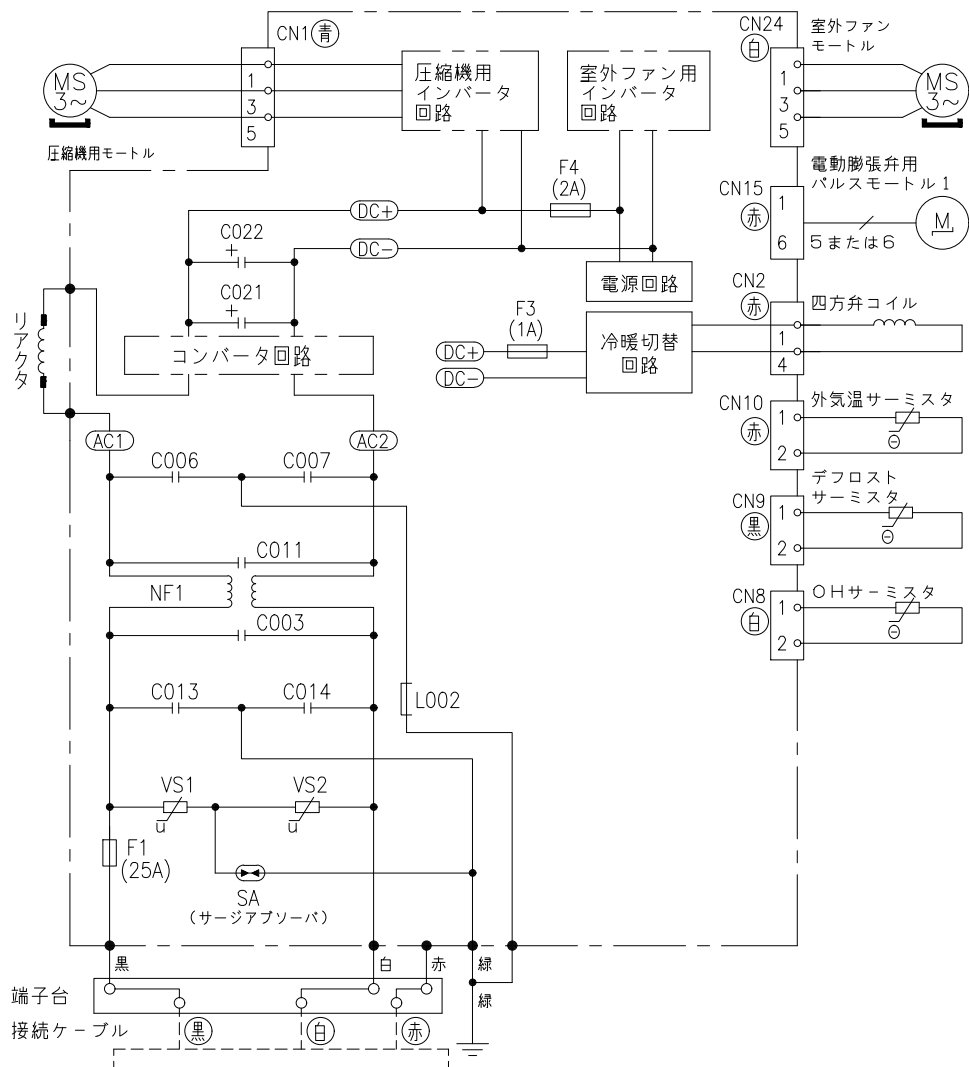
配線図 RAC-VL63K2EE
