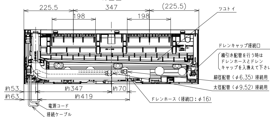
背面図
