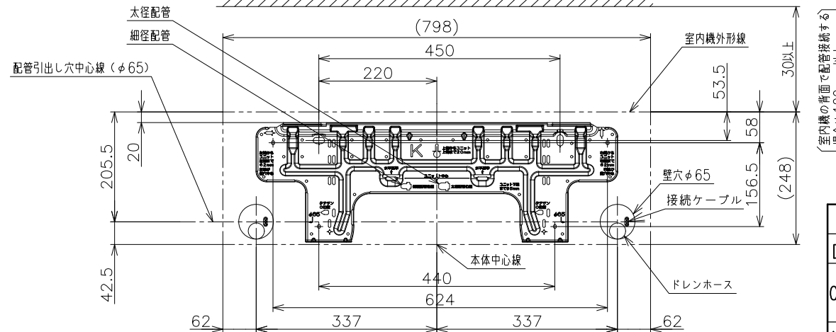
据付板 (正面図)
