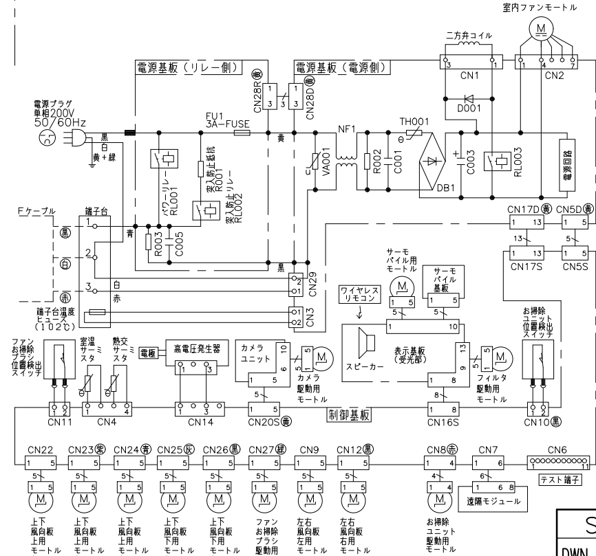
配線図 RAS-JT80K2SE8
