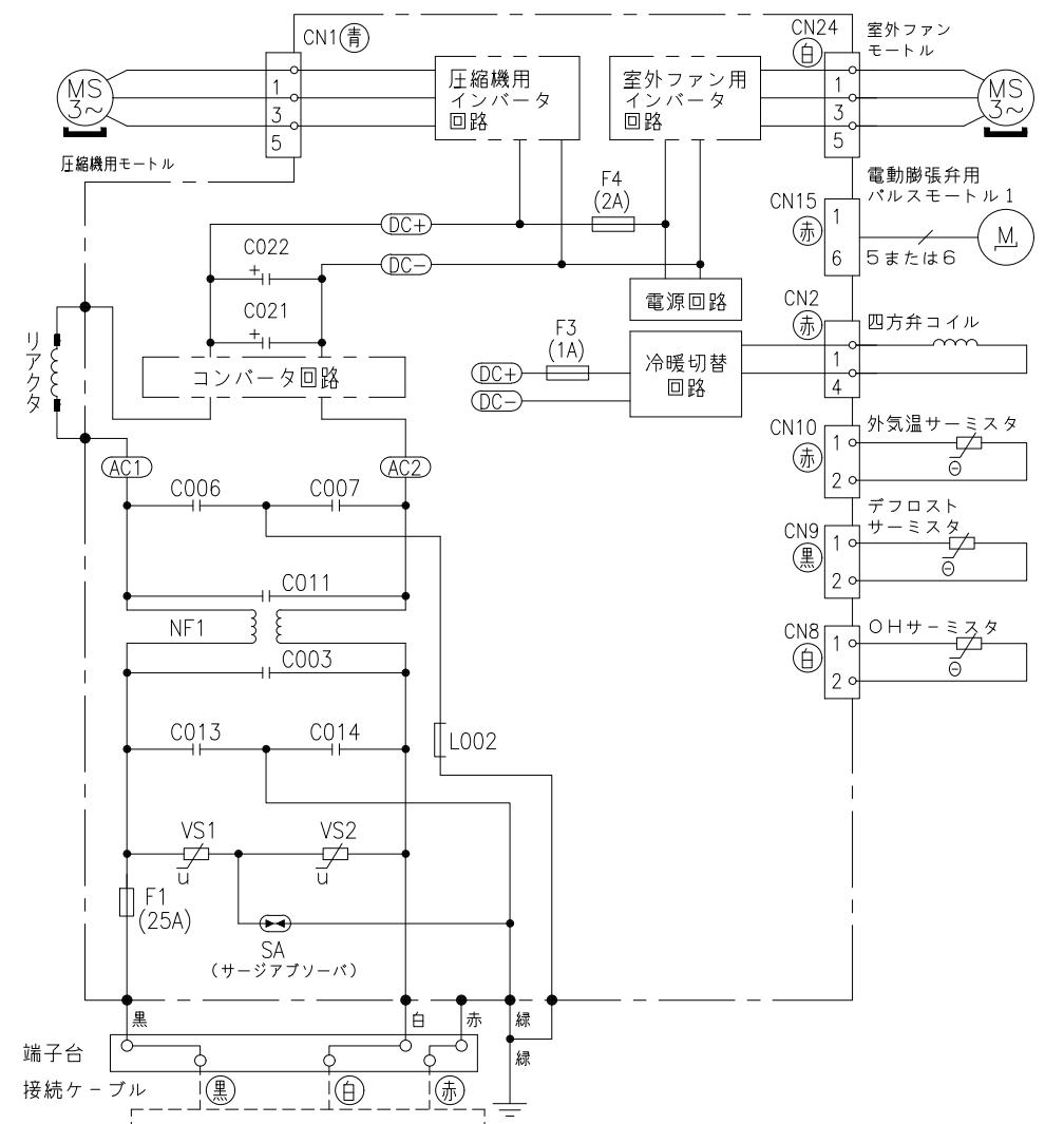
配線図 RAC-JT80K2SE8
