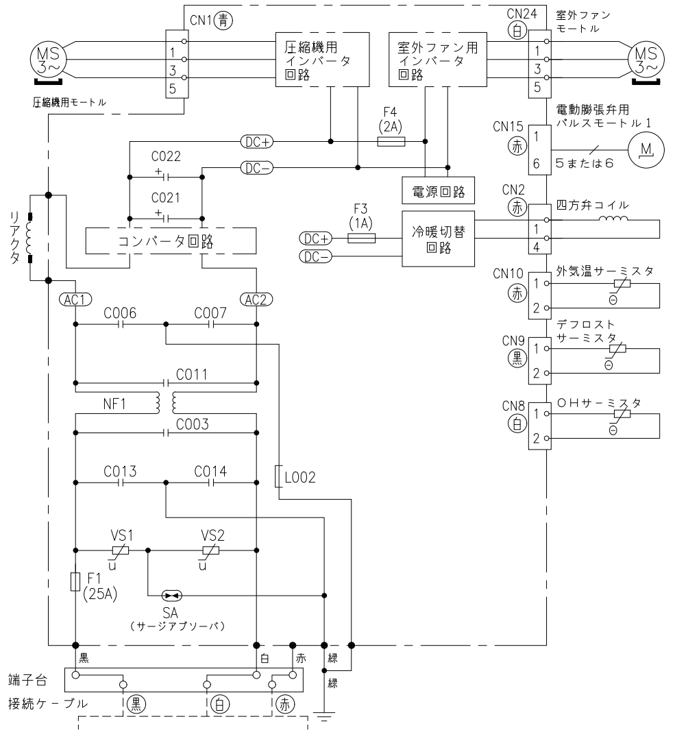
配線図 RAC-JT71K2SE8
