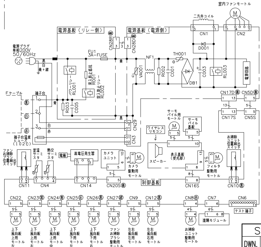
配線図 RAS-JT71K2SE8
