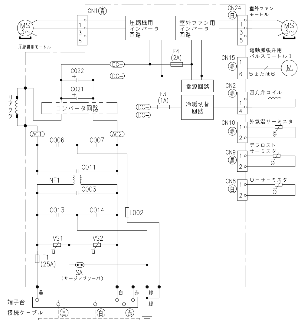
配線図 RAC-JT56K2SE8
