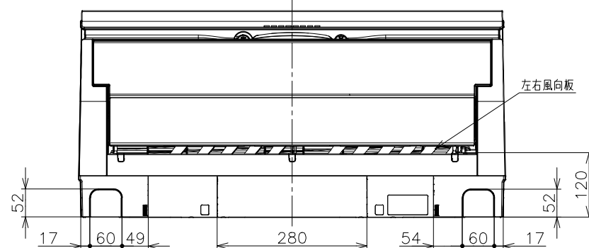
背面図
