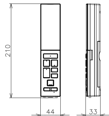
据付板
