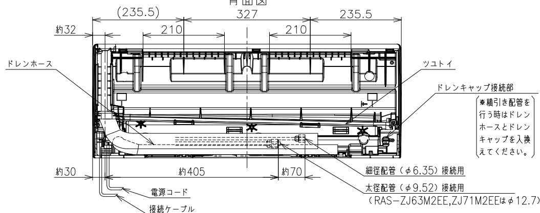
背面図
