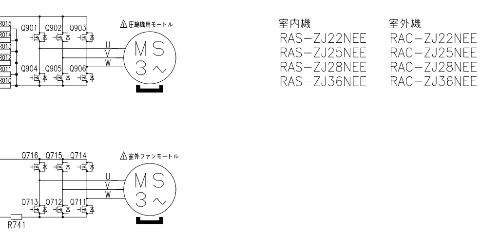
室外機配線図
