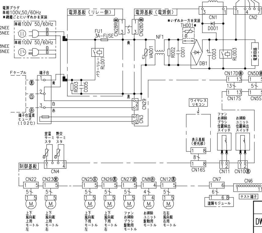
室内機配線図
