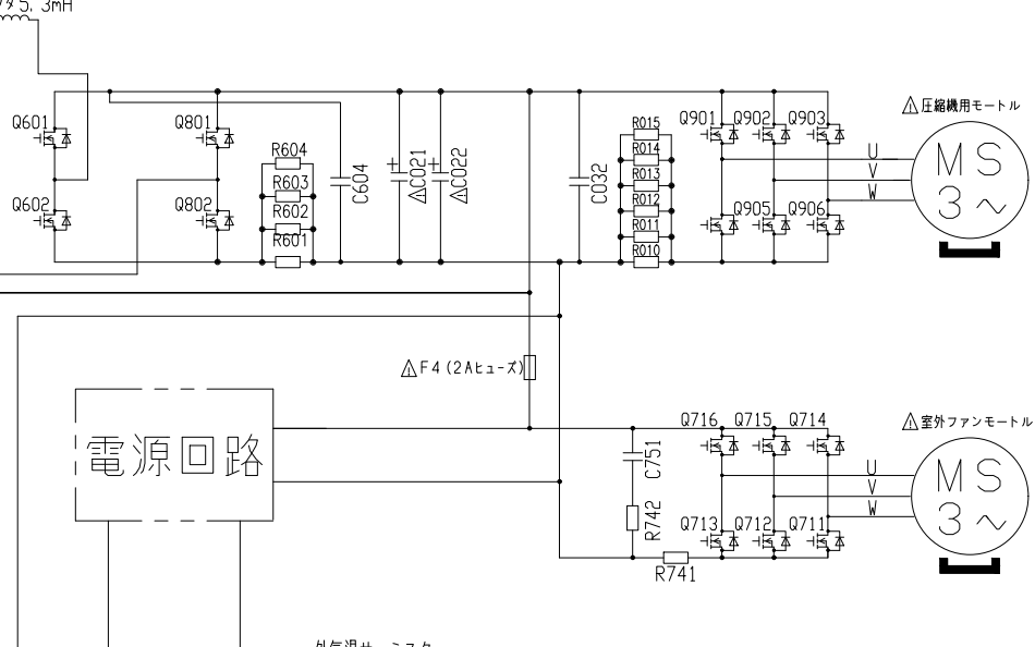
配線図 RAC-XJ90K2S
