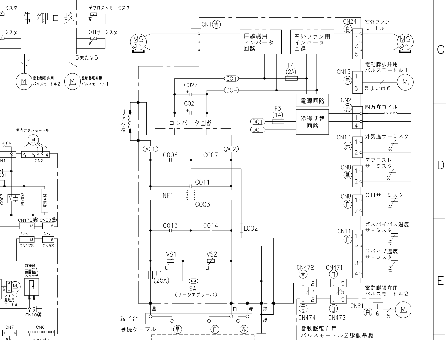
配線図 RAC-XJ90K2S
