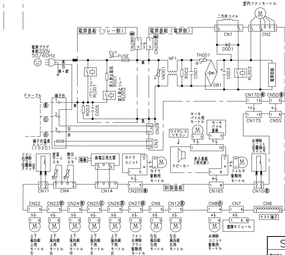
配線図 RAS-XJ90K2S
