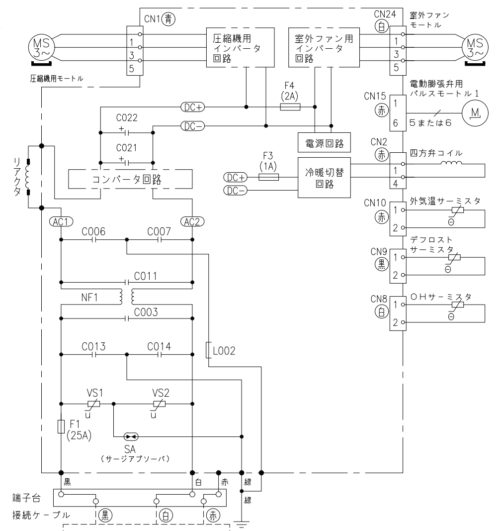
配線図 RAC-XJ80K2S
