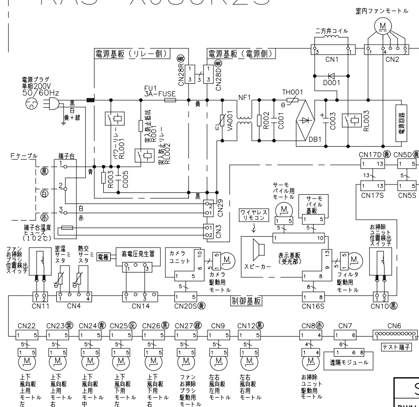
配線図 RAS-XJ80K2S
