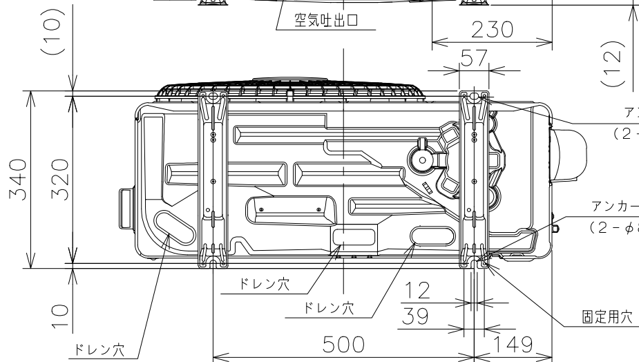
背面図
