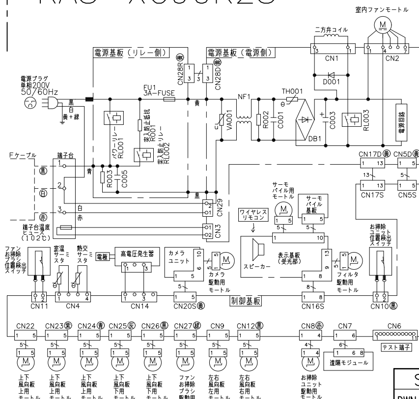
配線図 RAS-XC90K2S
