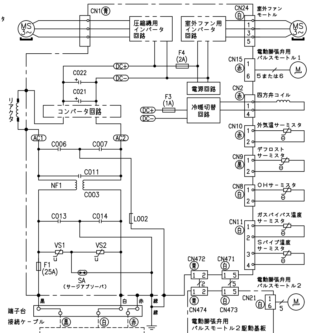
配線図 RAC-XC90K2S
