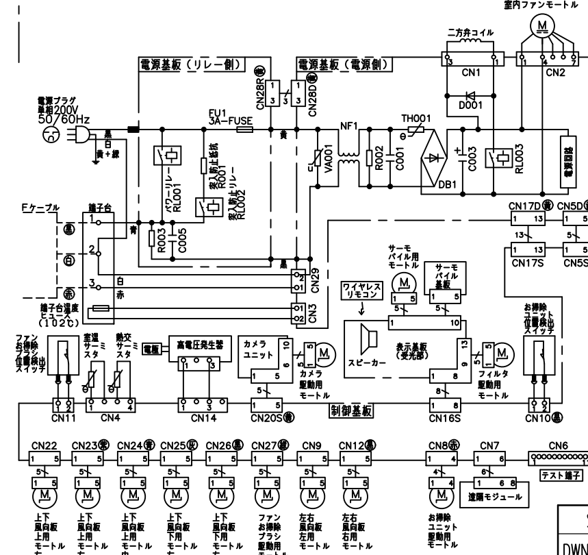
配線図 RAS-XC80K2S
