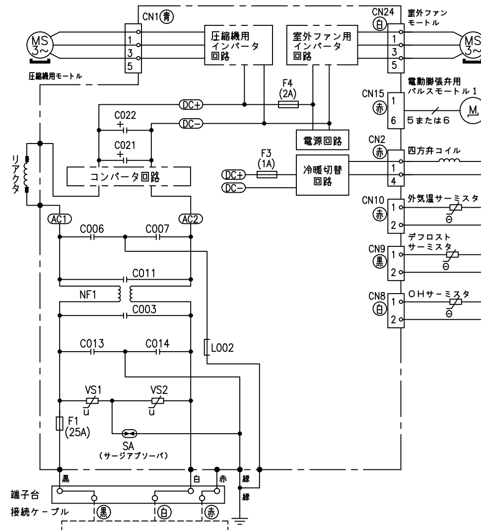
配線図 RAC-XC36K2S
