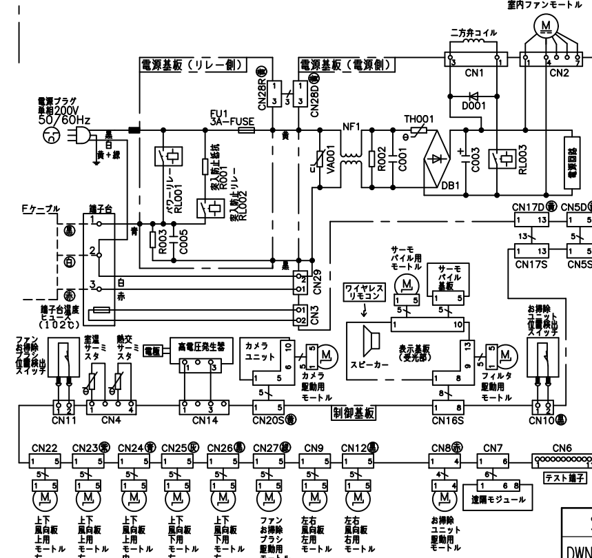
配線図 RAS-XC36K2S
