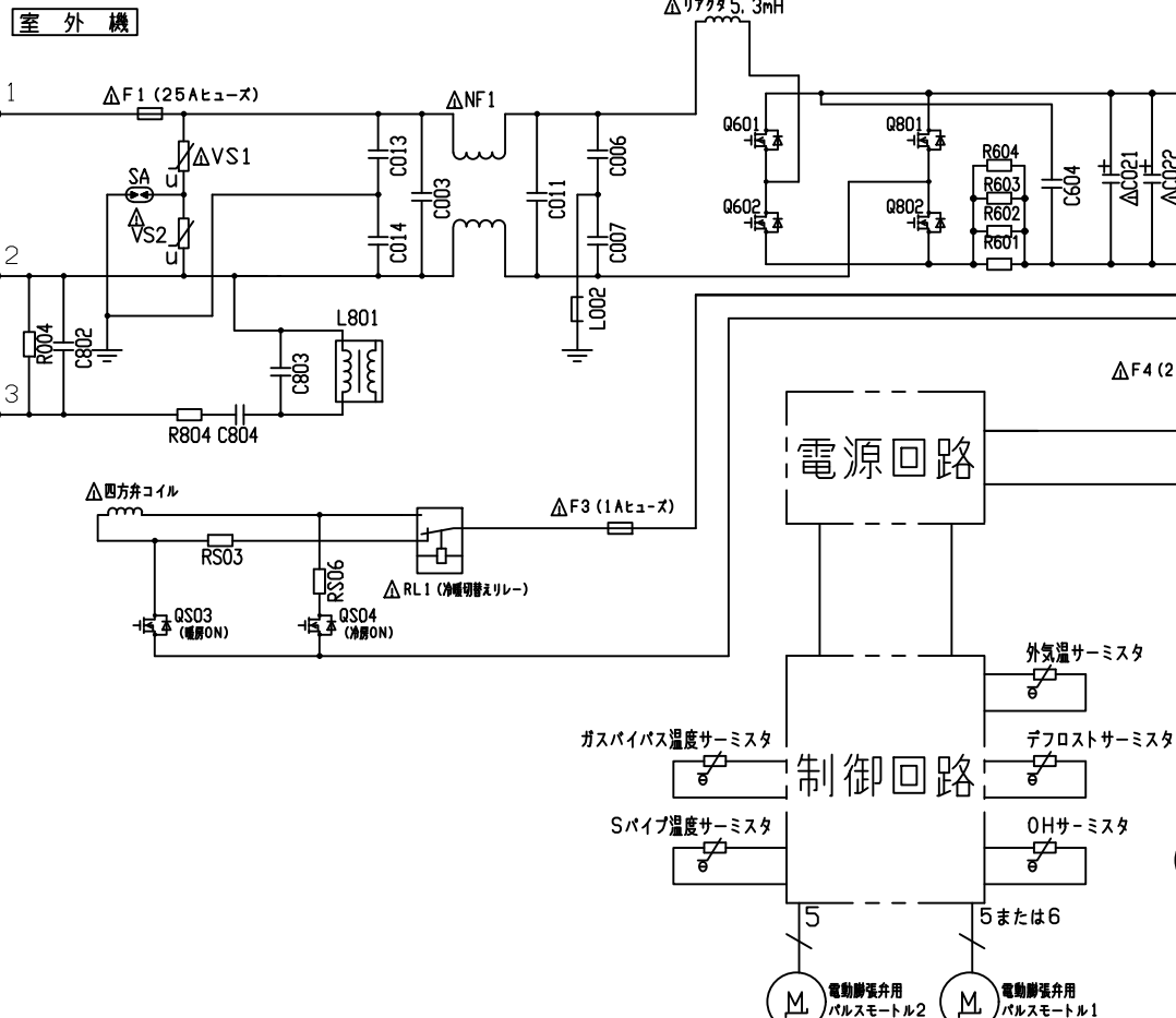
配線図 RAS-X90L2BK
