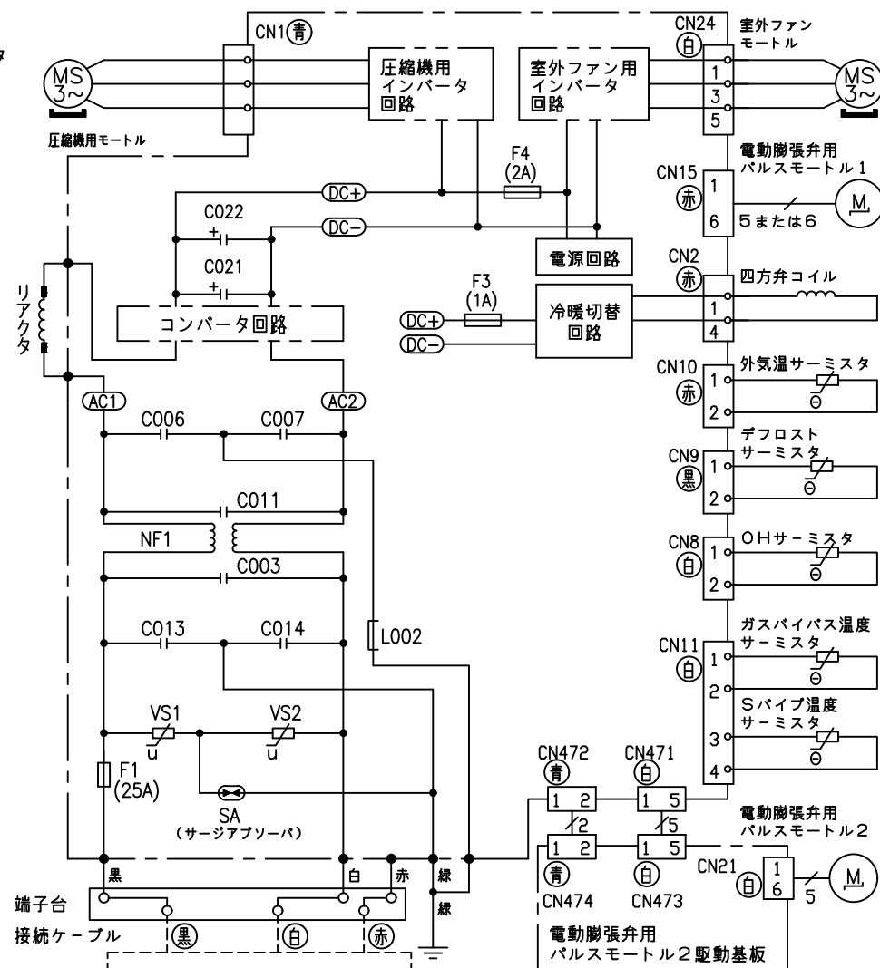
配線図 RAC-X90L2BK
