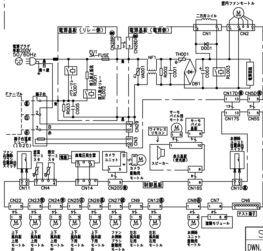
配線図 RAS-X90L2BK
