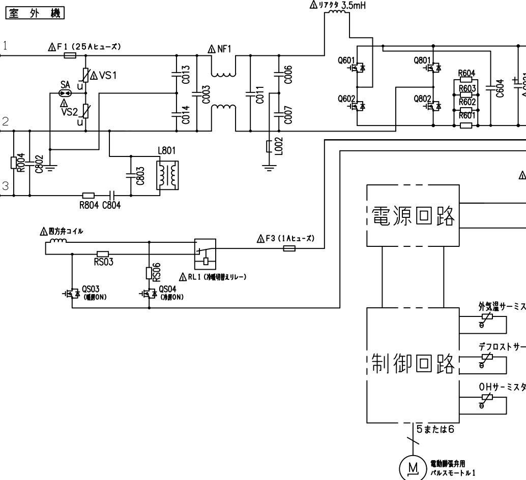
配線図 RAS-X80L2BK
