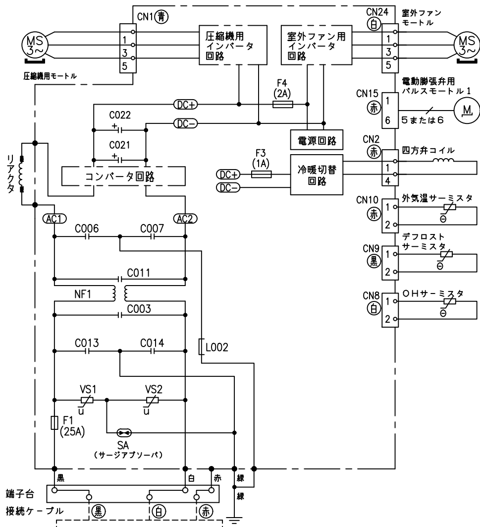
配線図 RAC-X80L2BK
