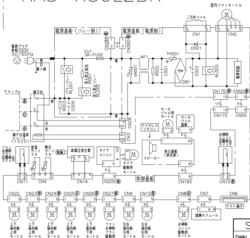
配線図 RAS-X80L2BK
