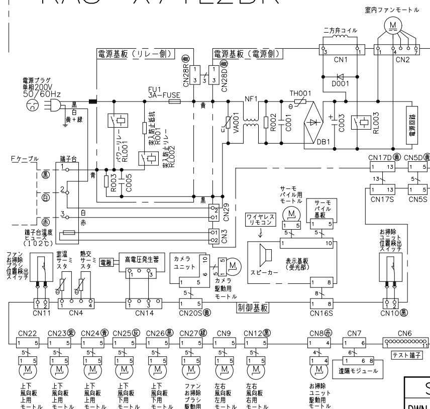
配線図 RAS-X71L2BK
