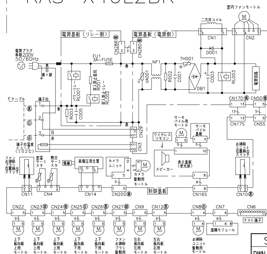
配線図 RAS-X40L2BK
