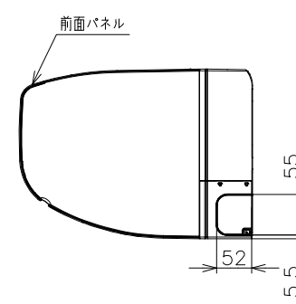
前面パネル
