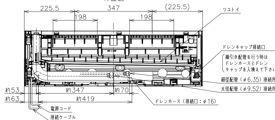
背面図
