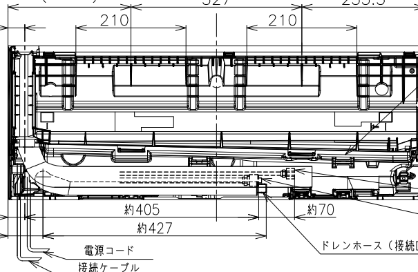
背面図
