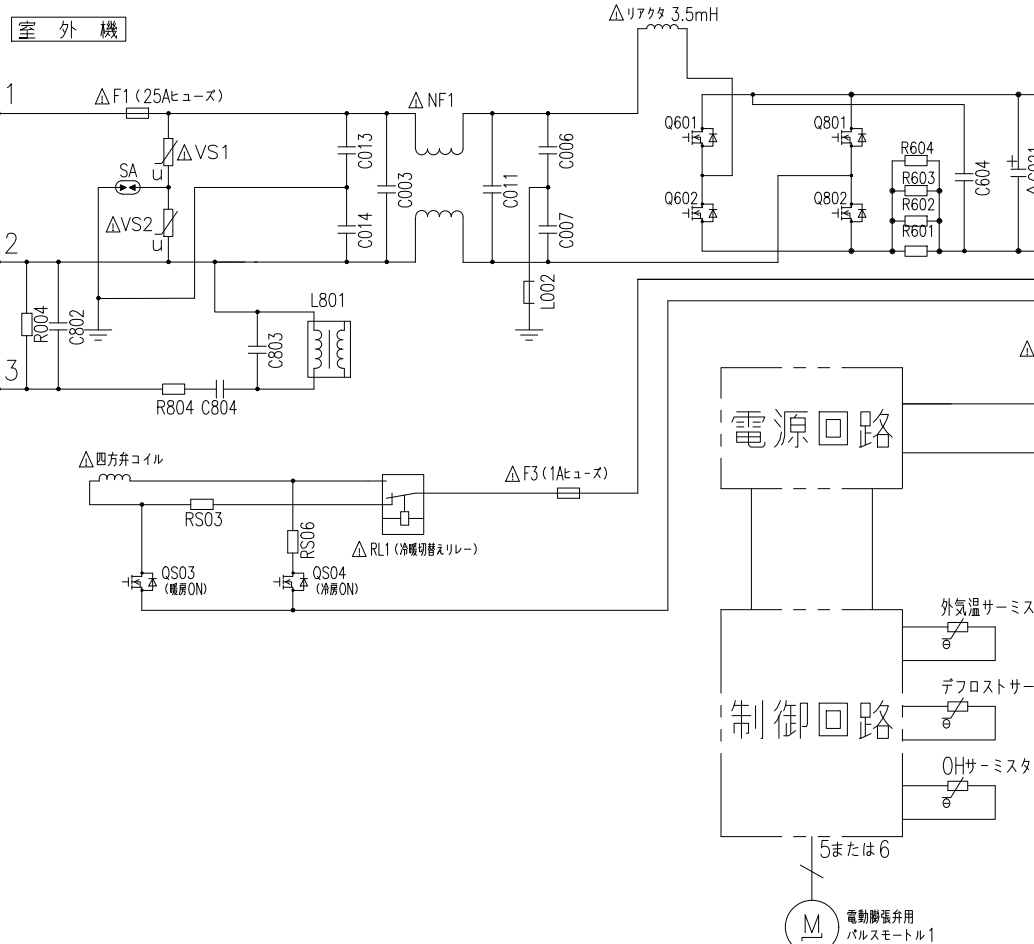
配線図 RAS-S63K2BK
