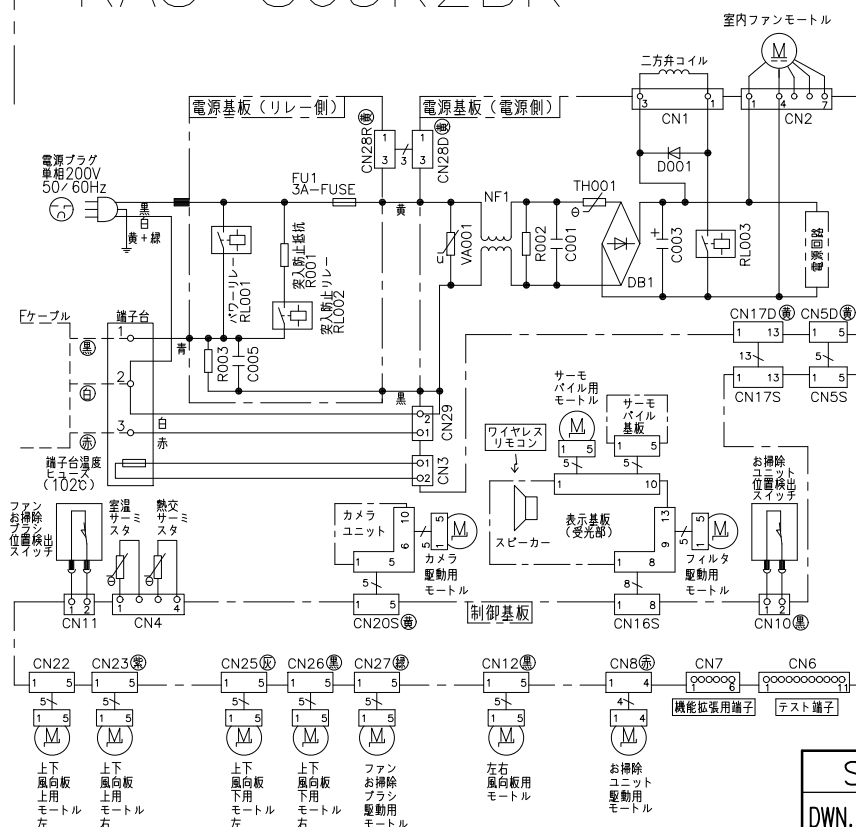
配線図 RAS-S63K2BK
