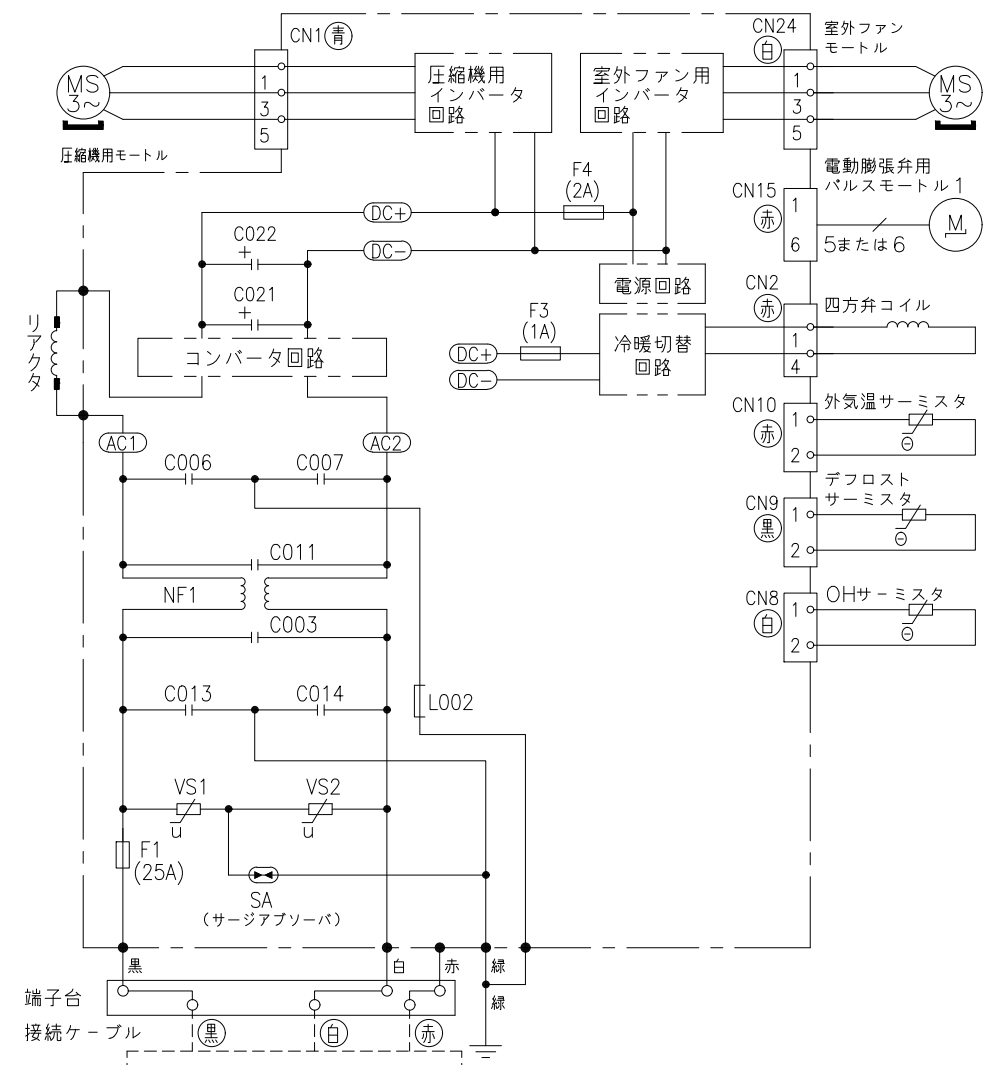
配線図 RAC-S63K2BK
