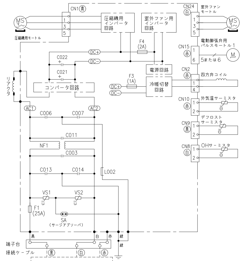
配線図 RAC-S56K2BK
