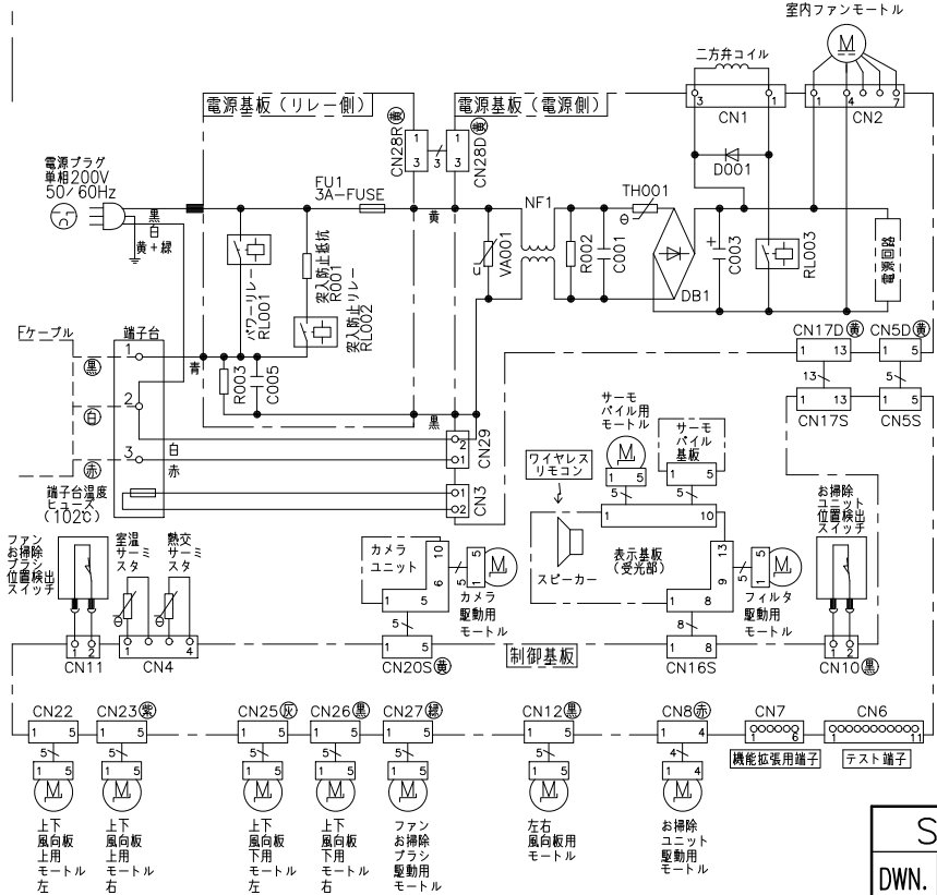
配線図 RAS-S56K2BK
