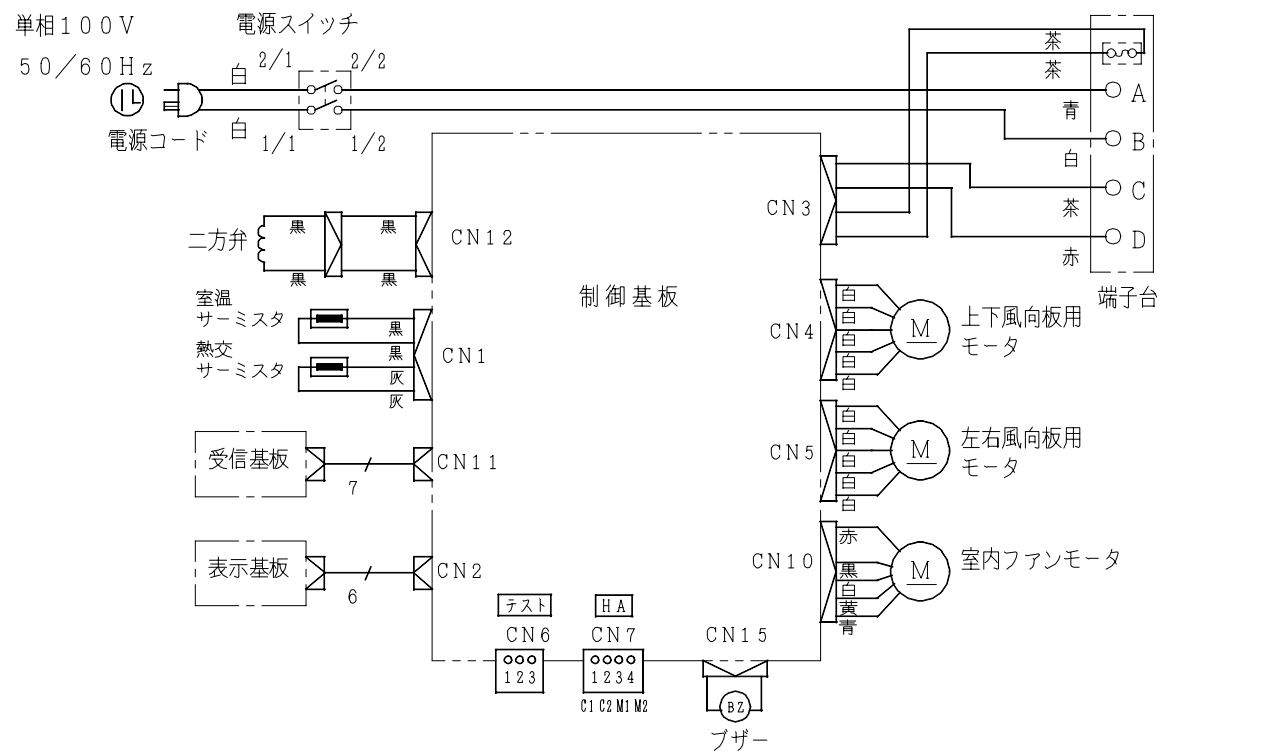
配線図 RAS-R2810KX
