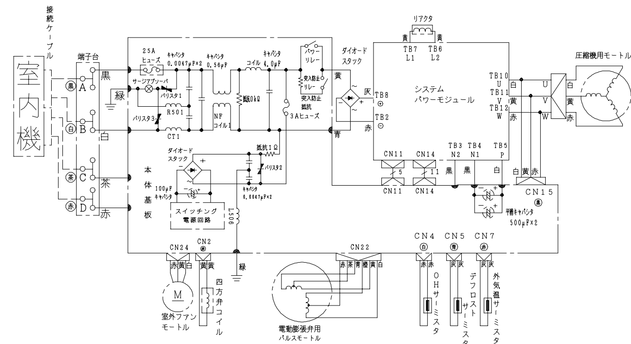
配線図 RAC-2810KX
