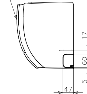
前面パネル
