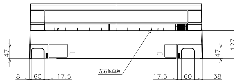
背面図
