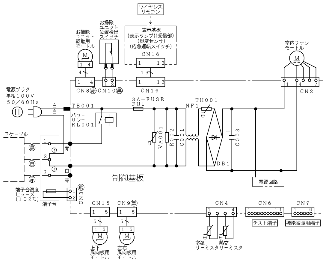
配線図 RAS-MJ25HEE
