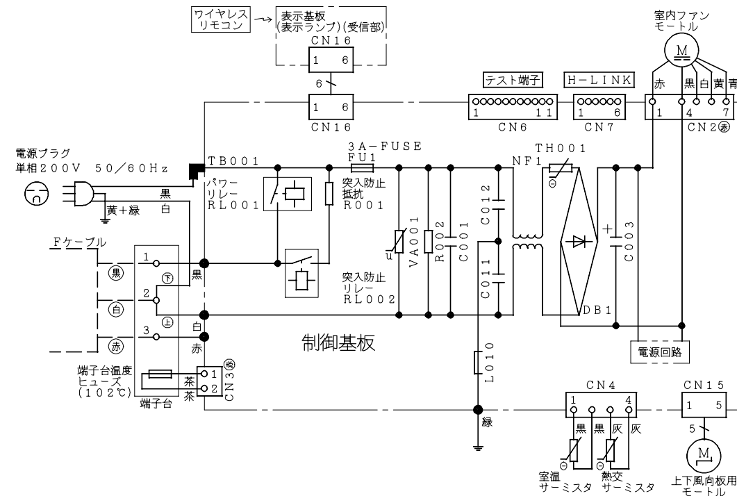
配線図 RAS-L40D2E2
