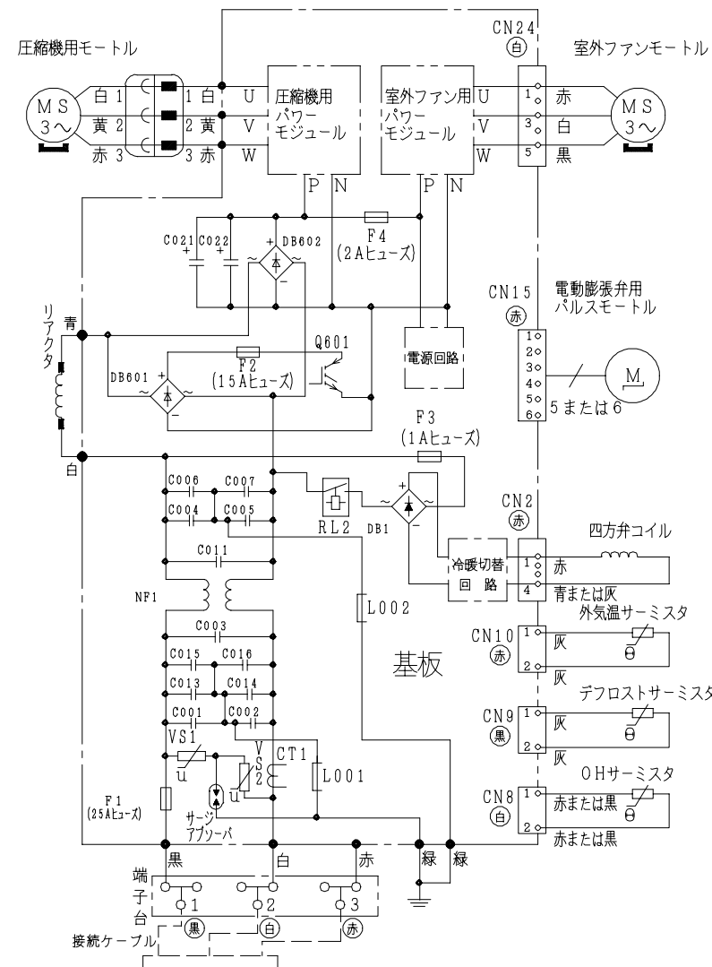
配線図 RAC-L40D2E2
