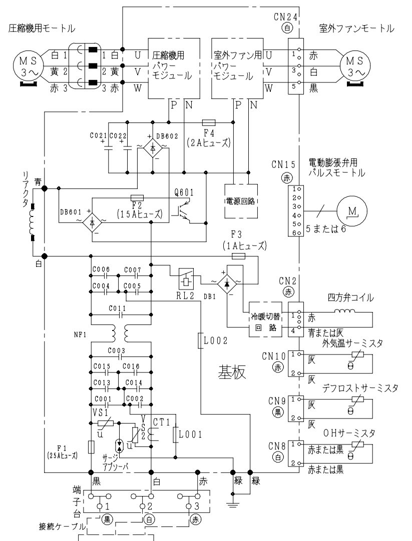
配線図 RAC-L40C2E1
