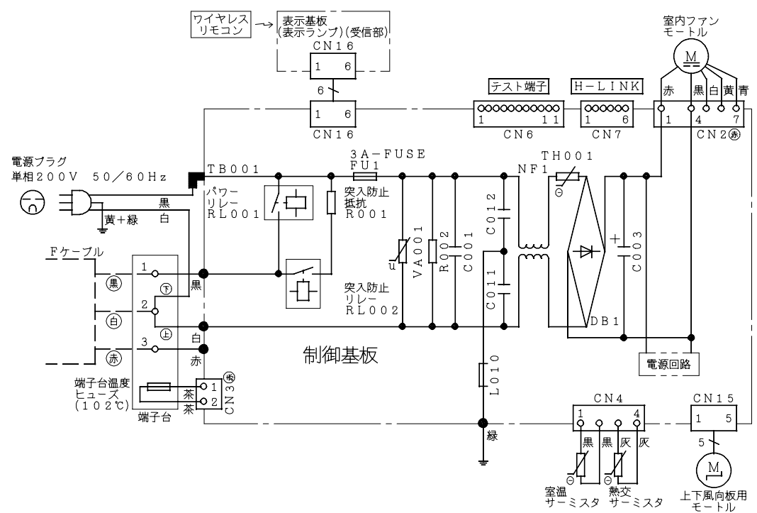
配線図 RAS-L40C2E1
