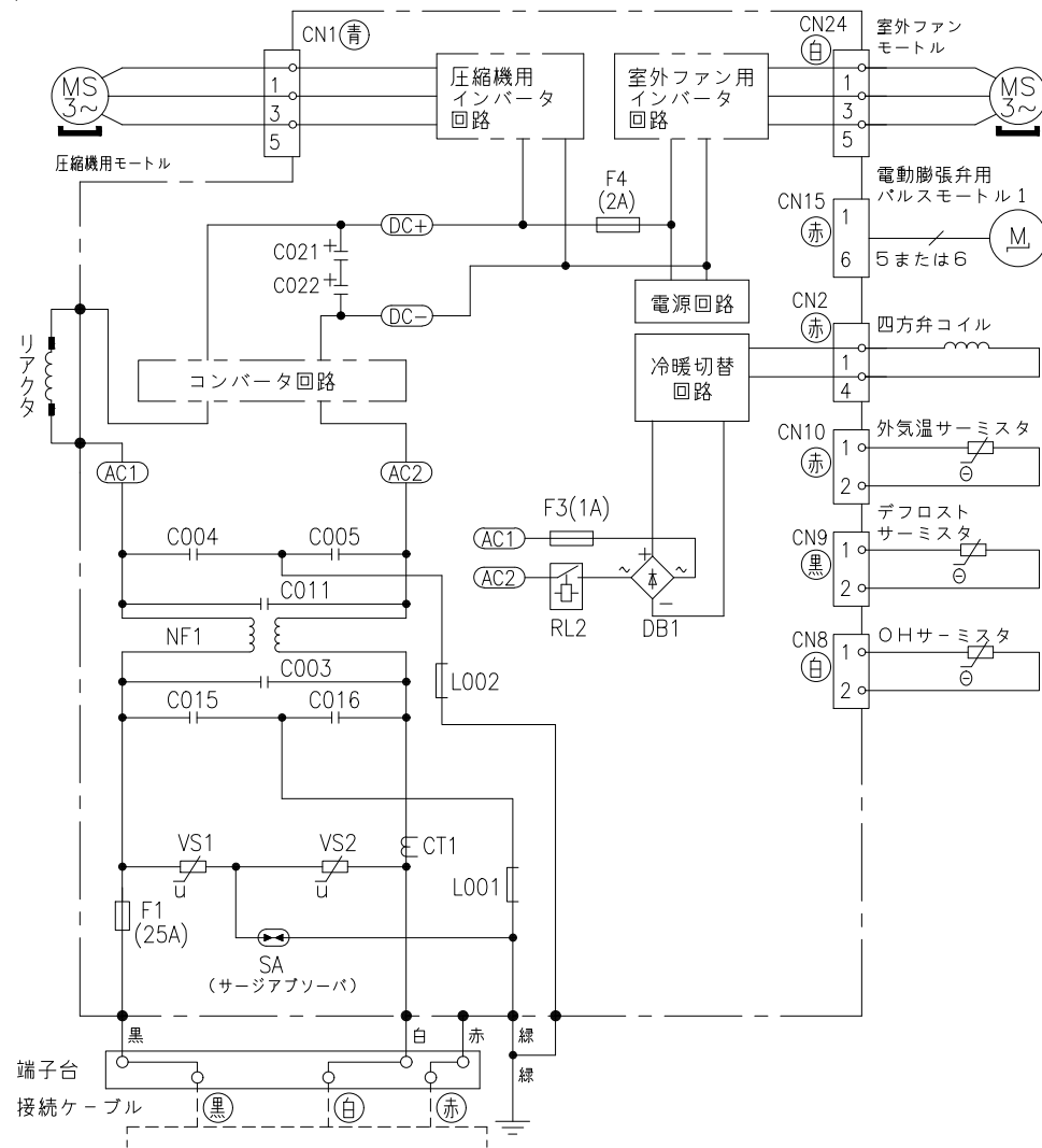
配線図 RAC-JT28KE8
