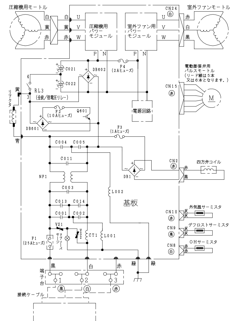
配線図 RAC-JT25ZE7
