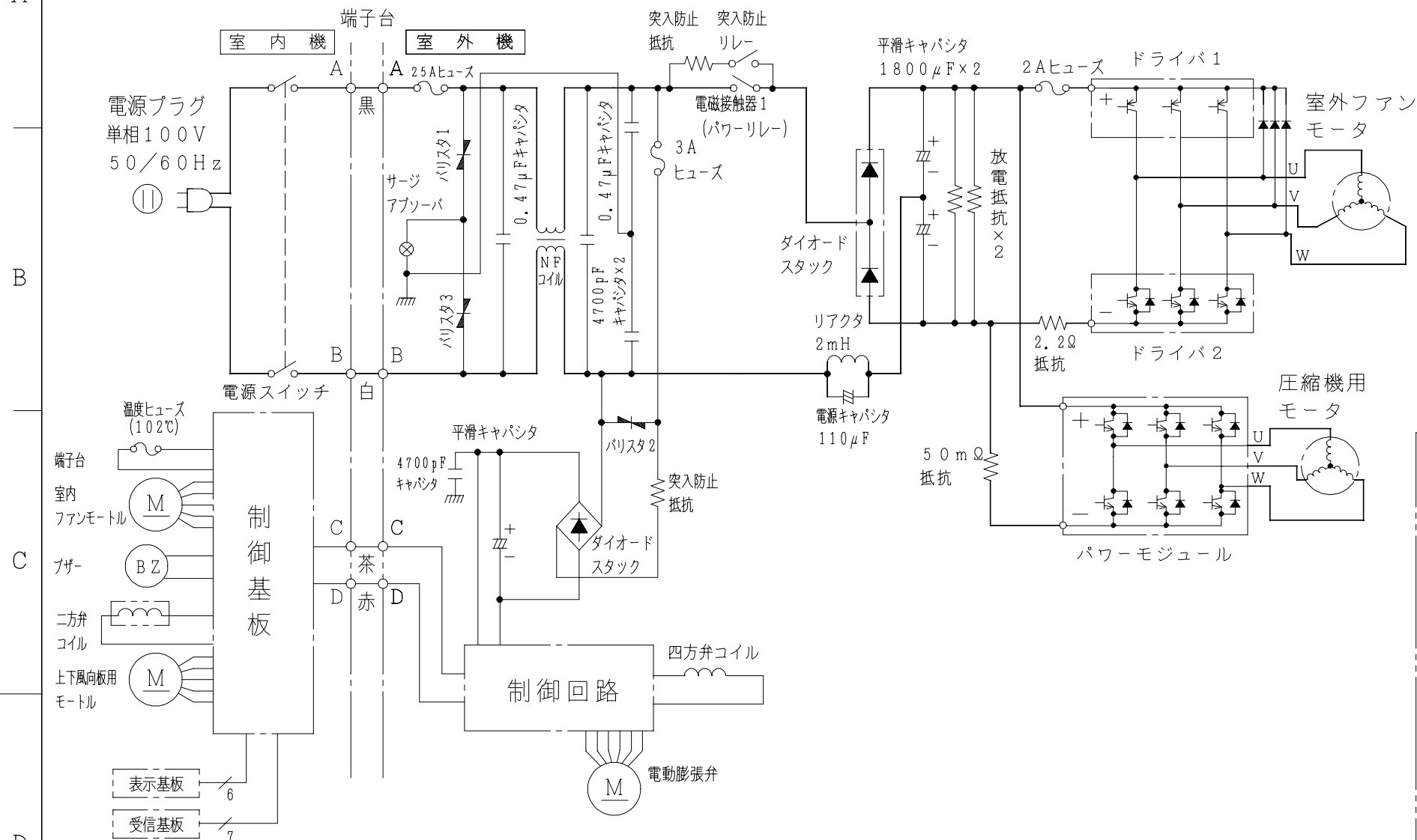
配線図 RAS-H2809LX
