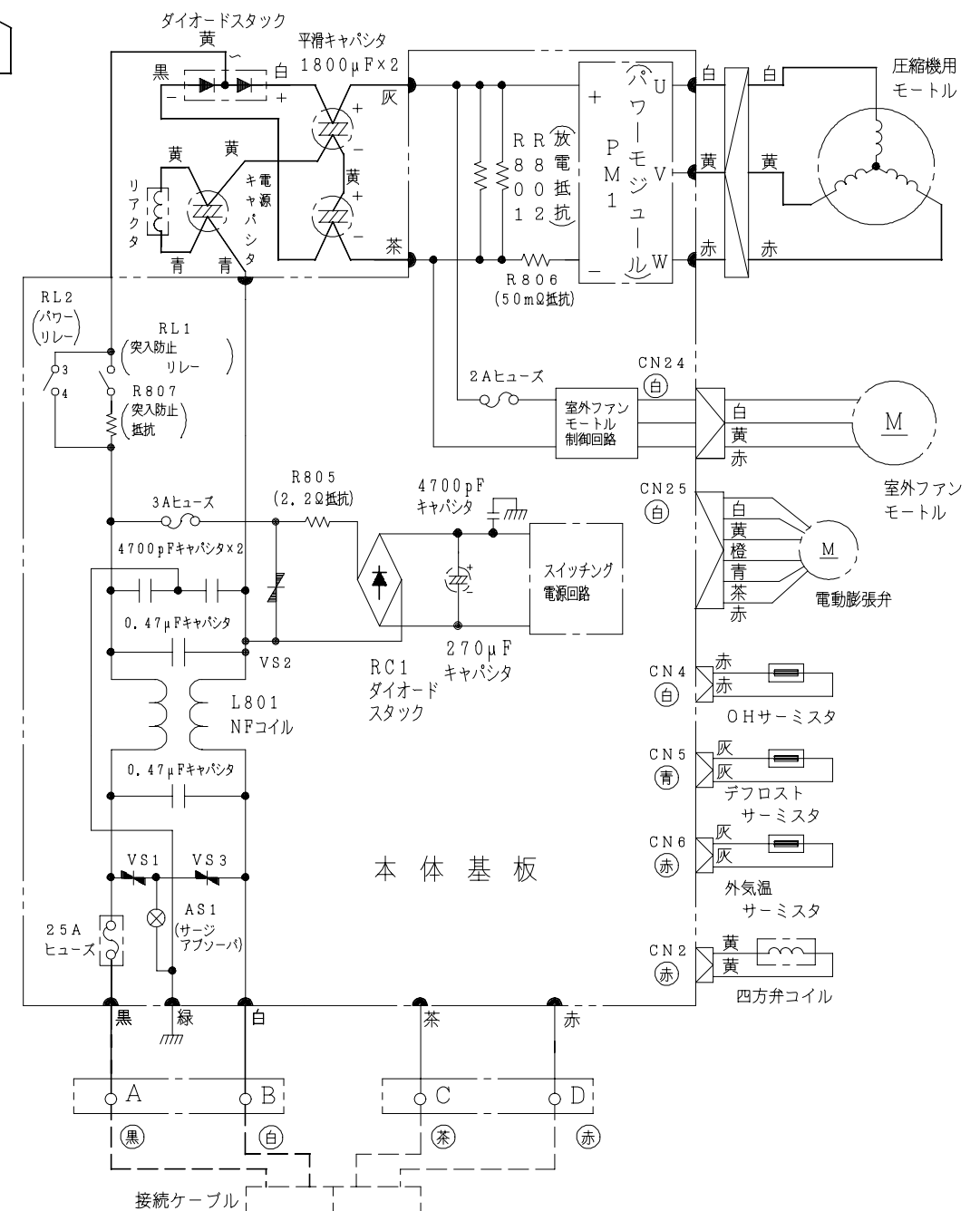
配線図 RAC-2809LX
