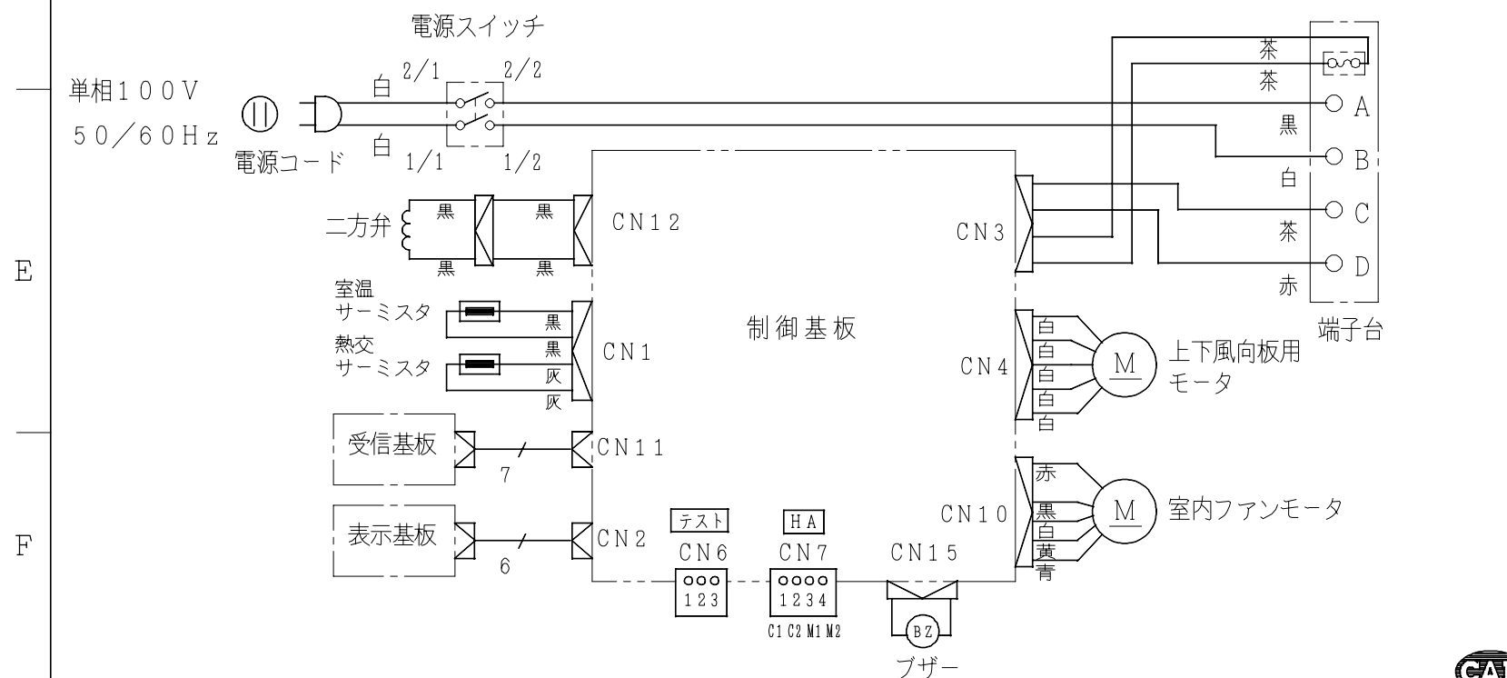
配線図 RAS-H2809LX
