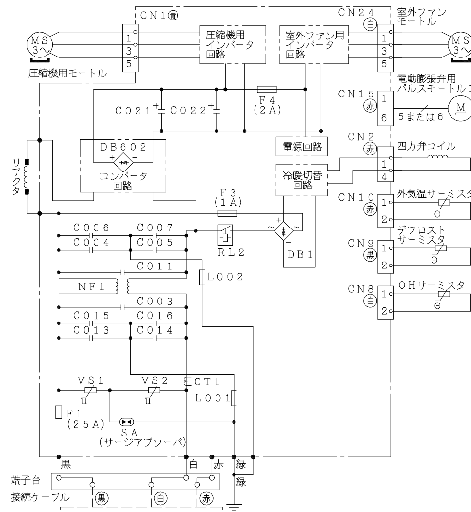
配線図 RAC-EBK40H2
