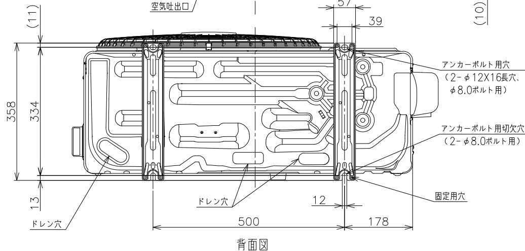
背面図
