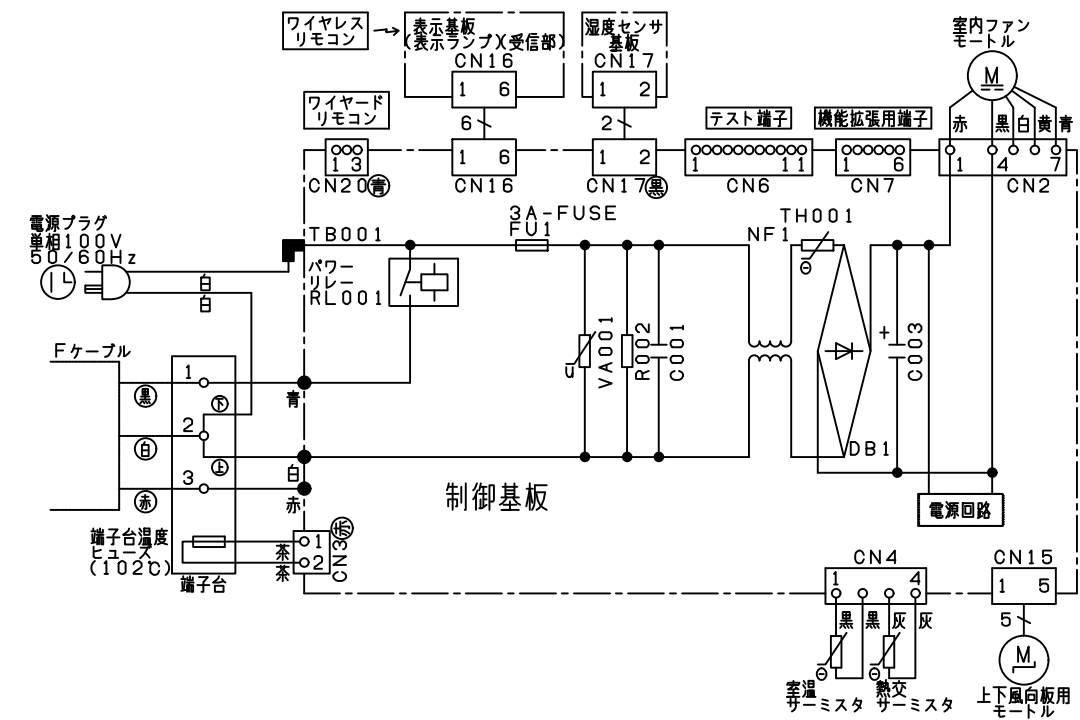
配線図 RAS-AJ40JEE
