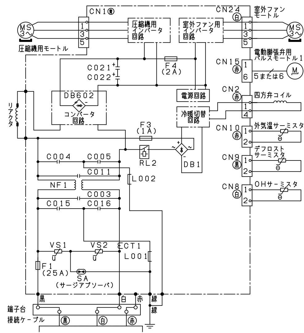
配線図 RAC-AJ40JEE
