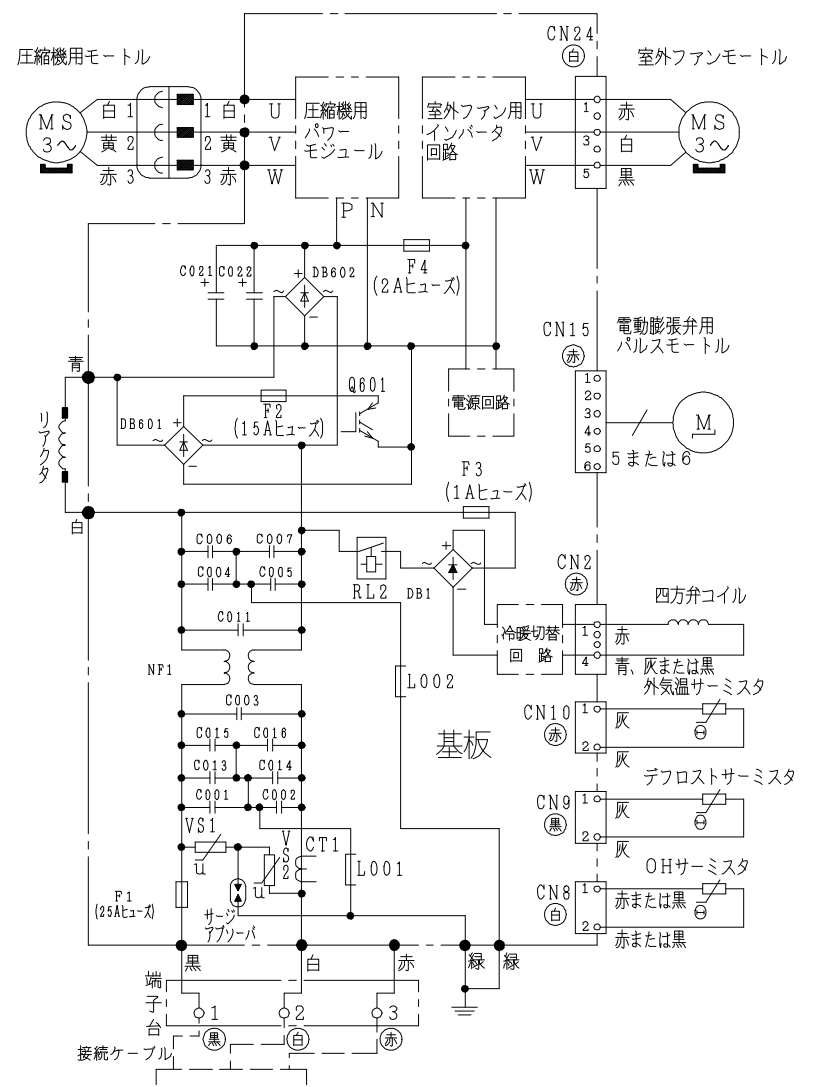
配線図 RAC-AJ40F2E
