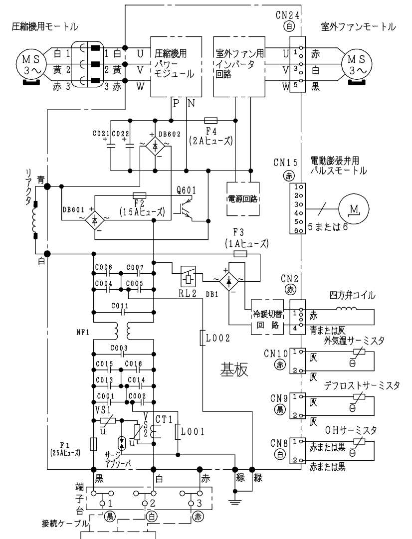
配線図 RAC-AJ40E2E
