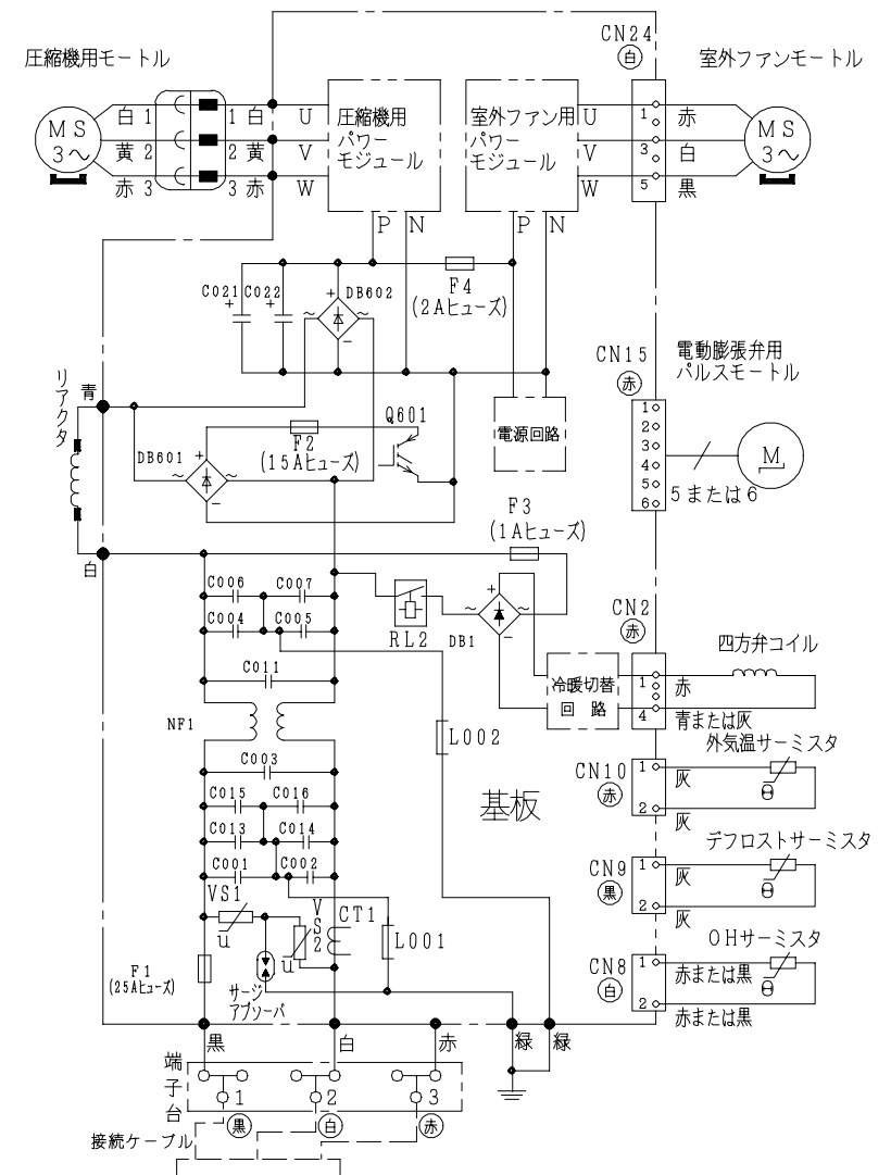
配線図 RAC-AJ40B2E
