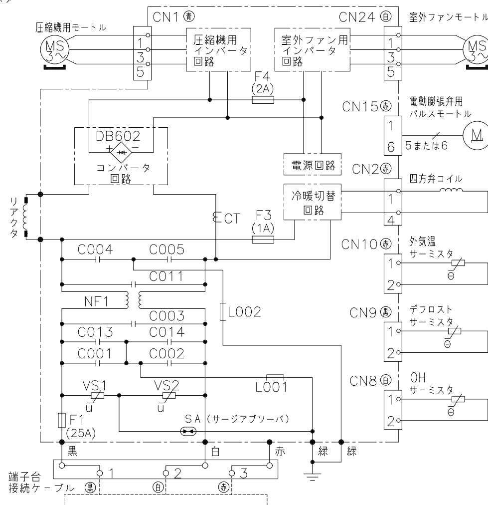
配線図 RAC-AJ36KEE
