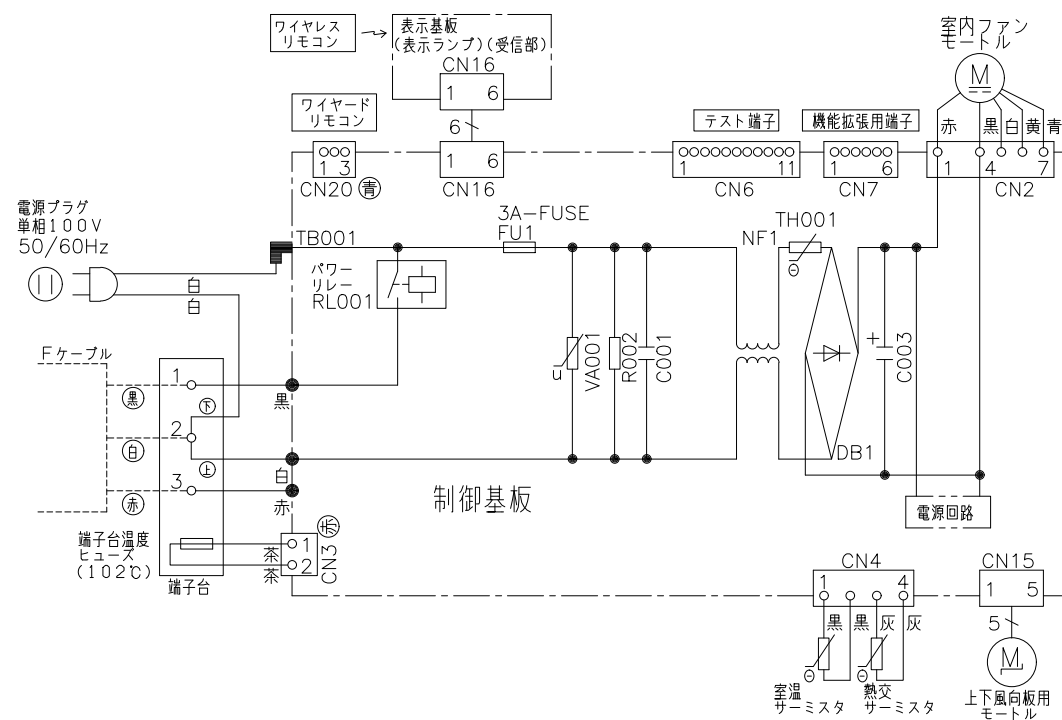
配線図 RAS-AJ36KEE
