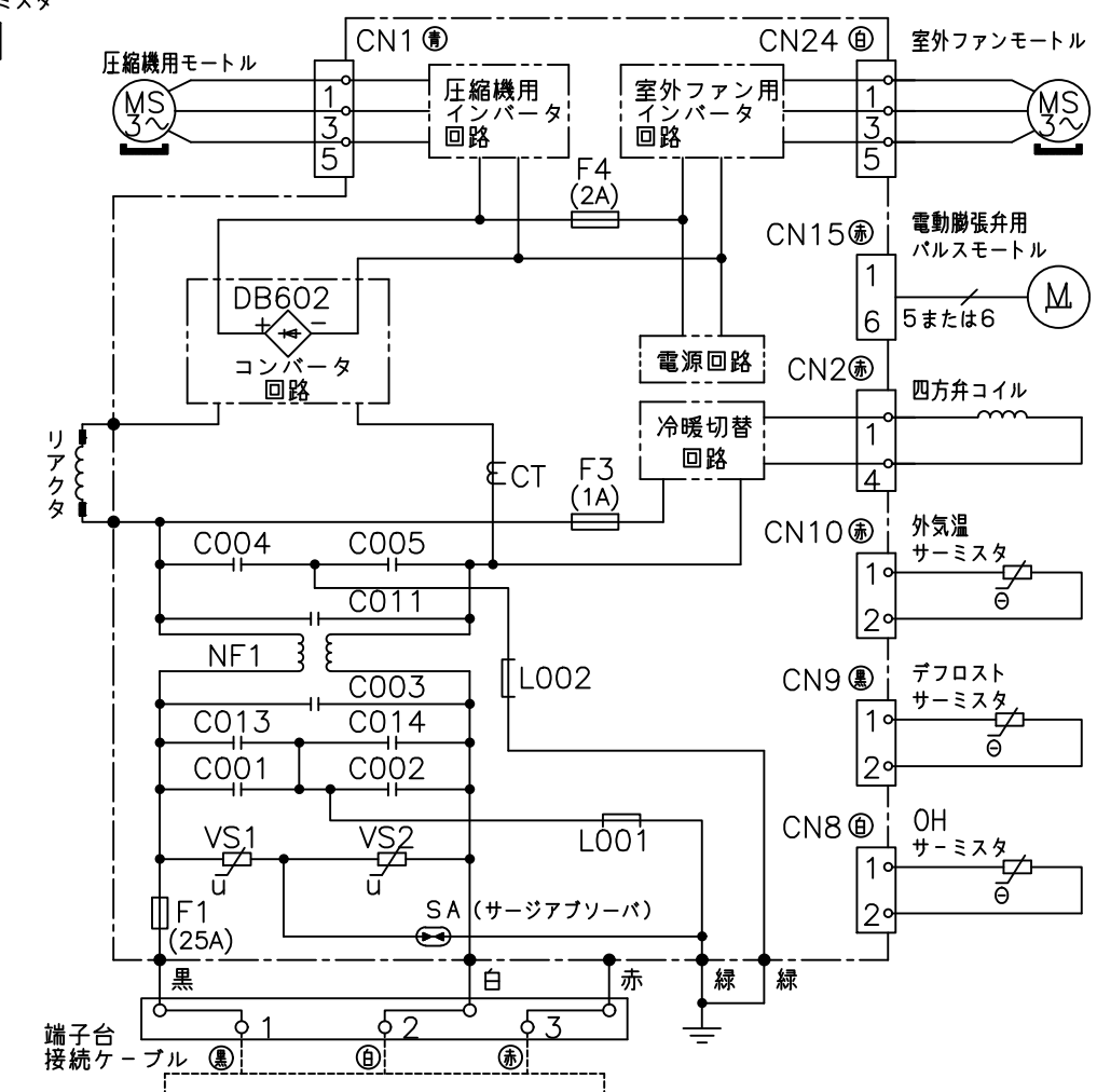
配線図 RAC-AJ36JEE
