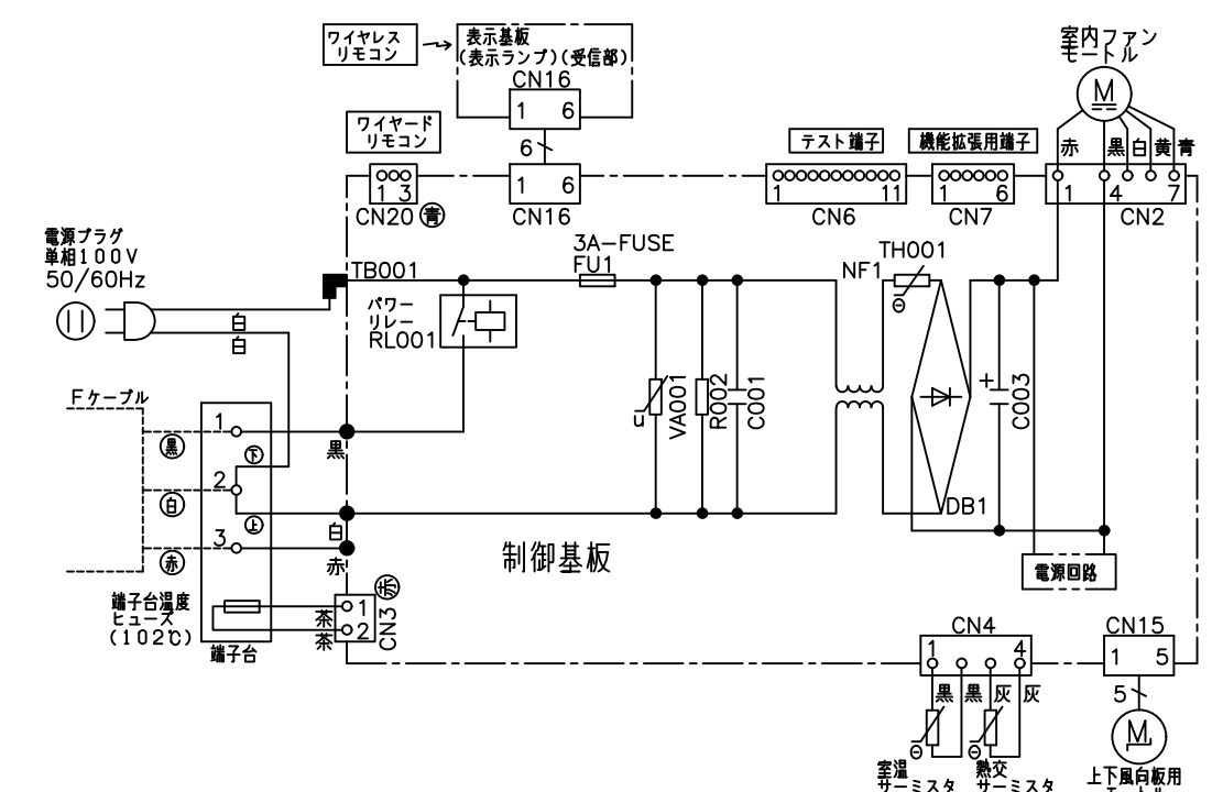
配線図 RAS-AJ36JEE
