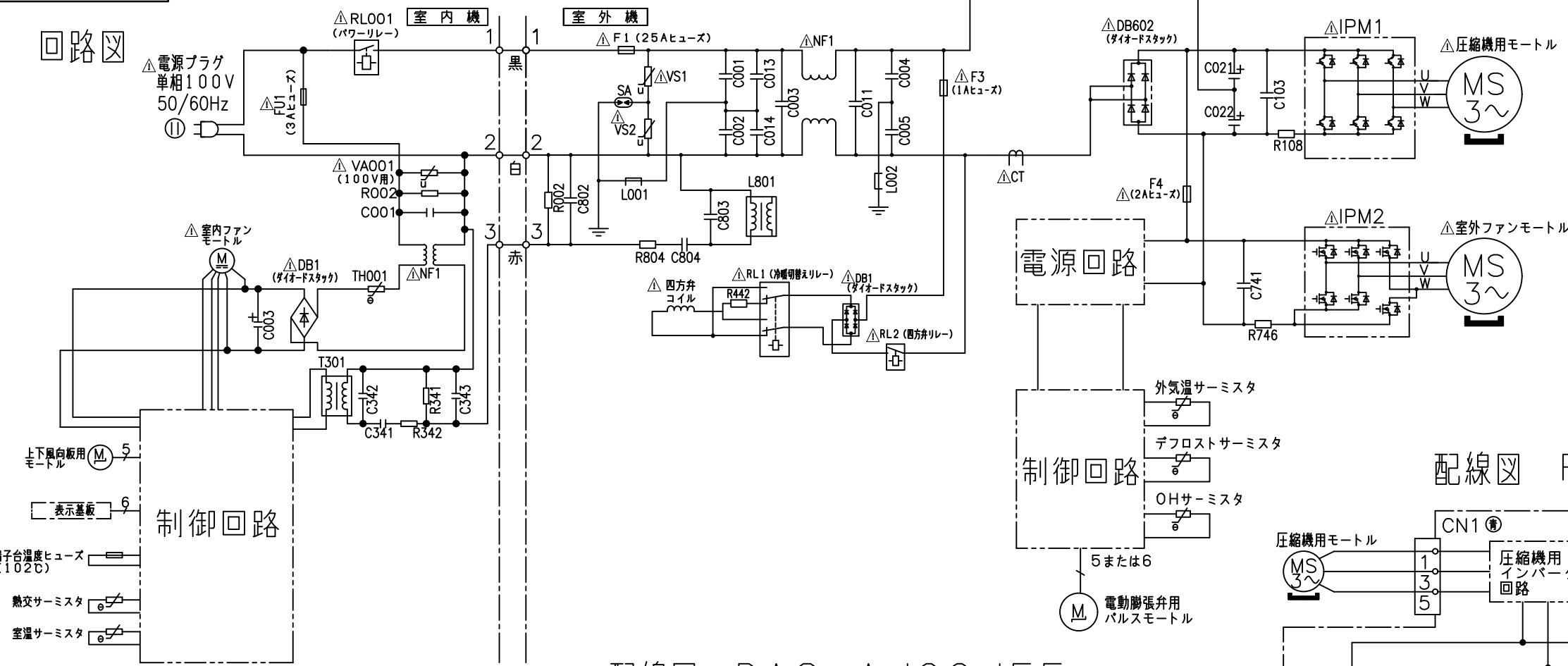
配線図 RAS-AJ36JEE
