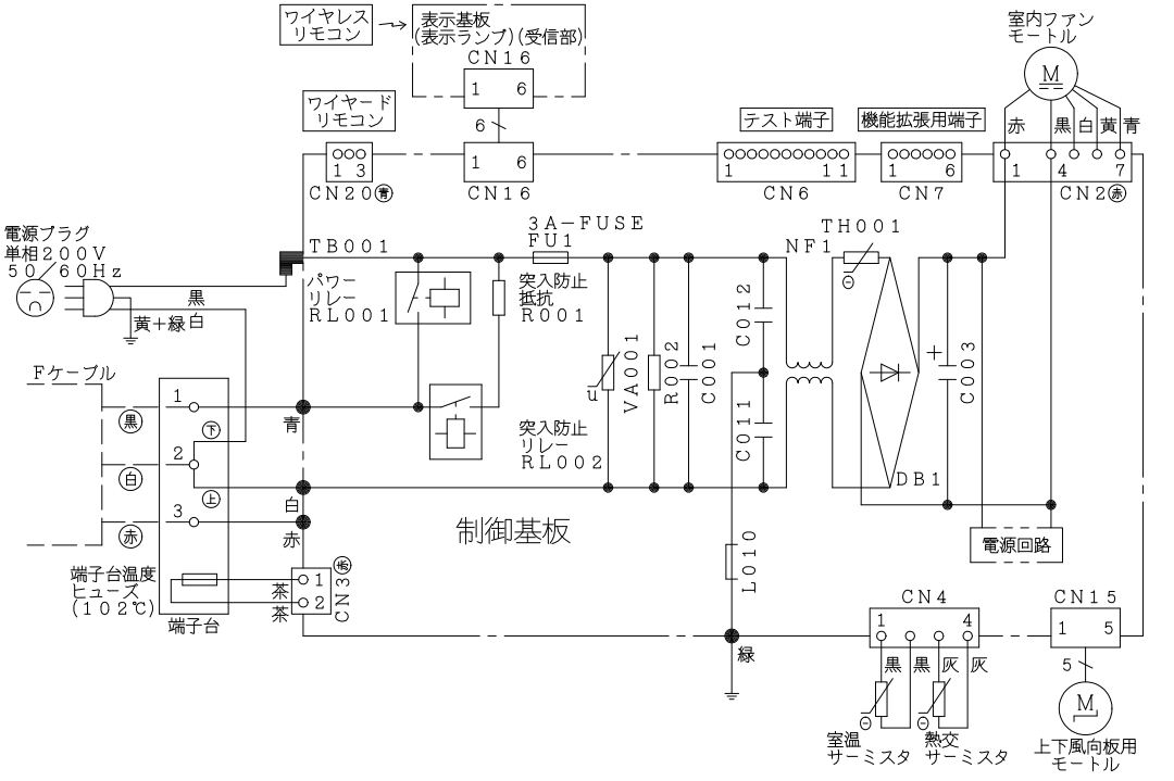
配線図 RAS-AJ36H2E
