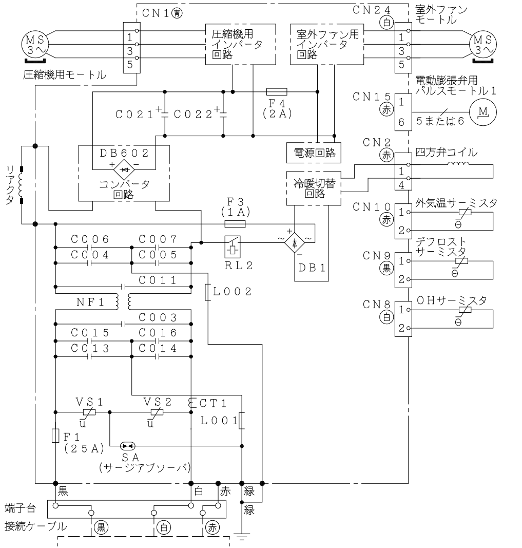
配線図 RAC-AJ36H2E
