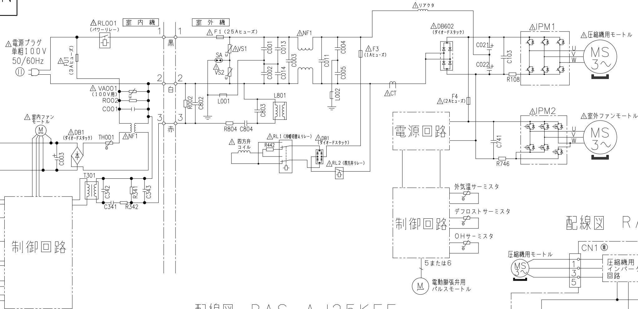
配線図 RAS-AJ25KEE
