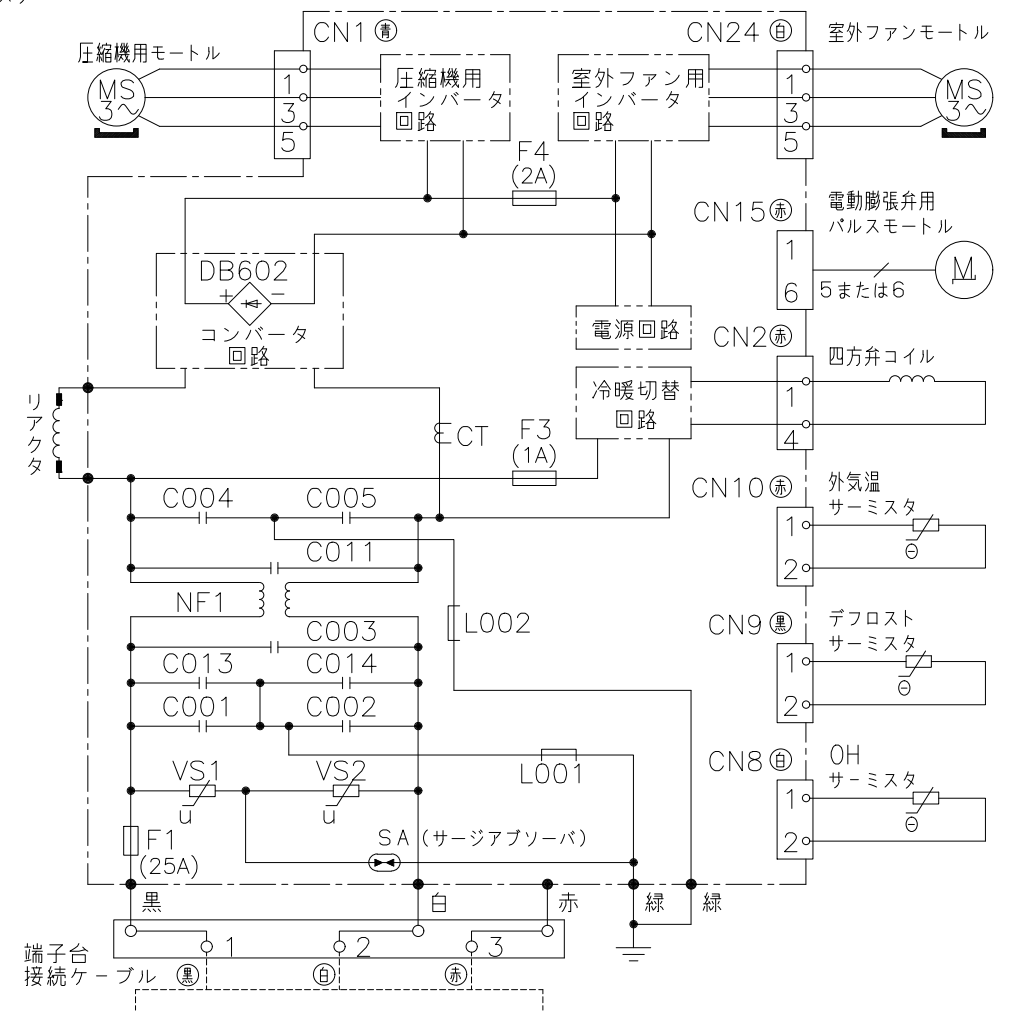
配線図 RAC-AJ25KEE
