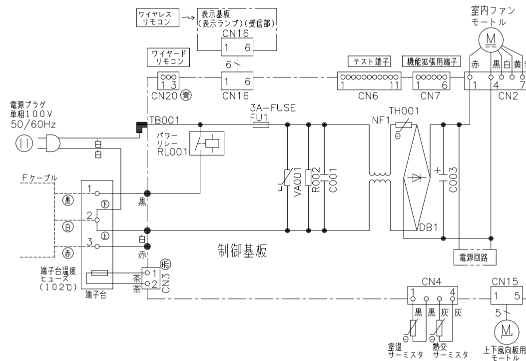
配線図 RAS-AJ25KEE
