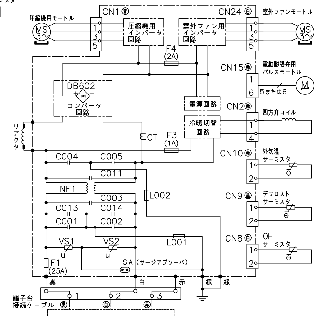
配線図 RAC-AJ25JEE
