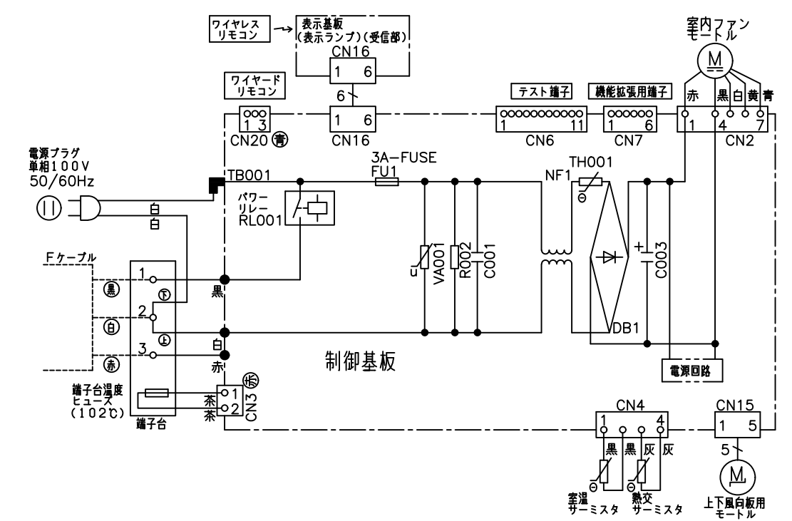
配線図 RAS-AJ25JEE
