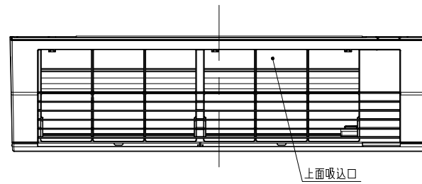
日立ルームエアコン 壁掛A Jシリーズ 室内ユニット寸法図
