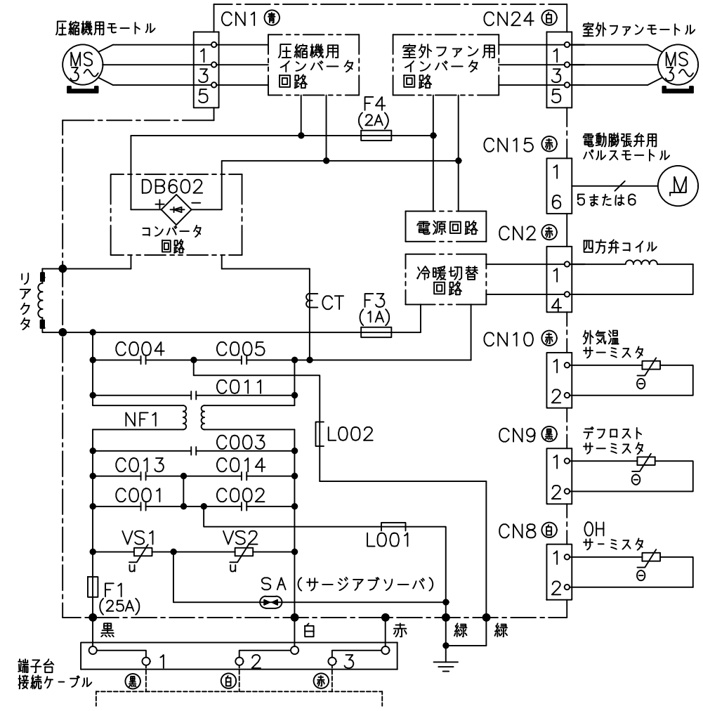
配線図 RAC-AJ22JEE
