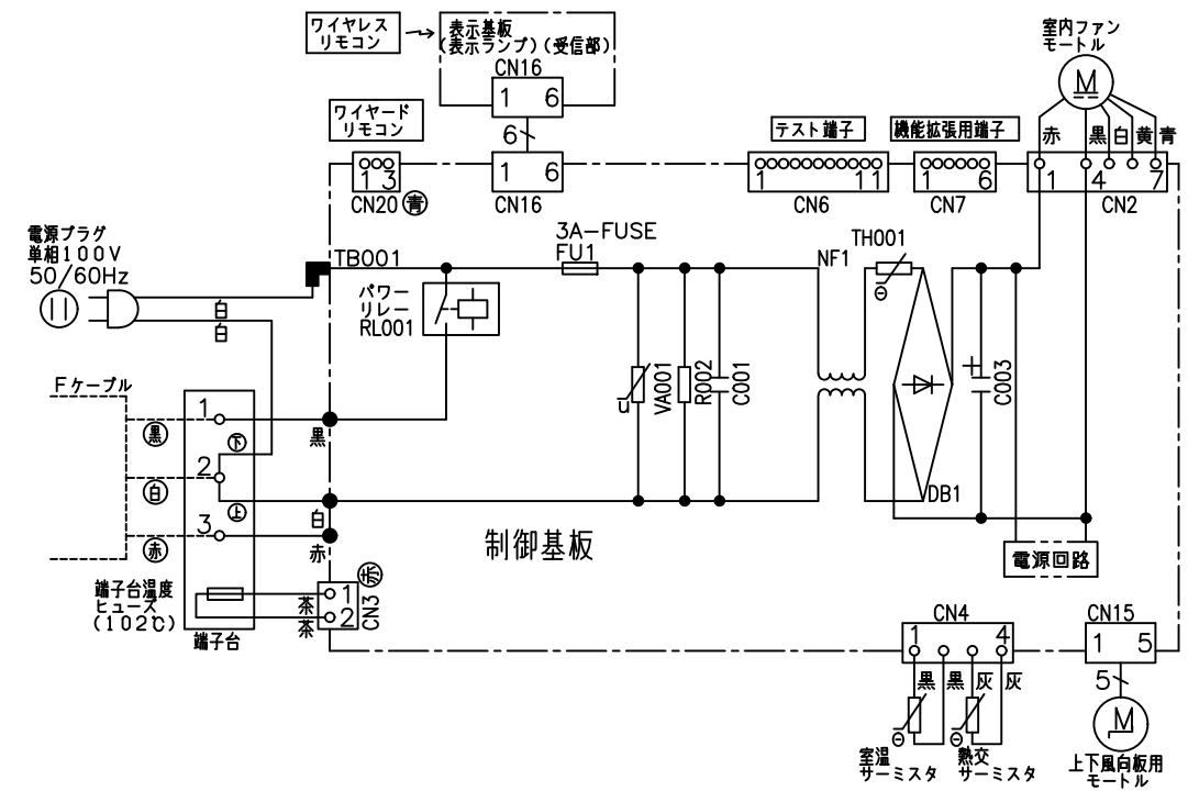
配線図 RAS-AJ22JEE
