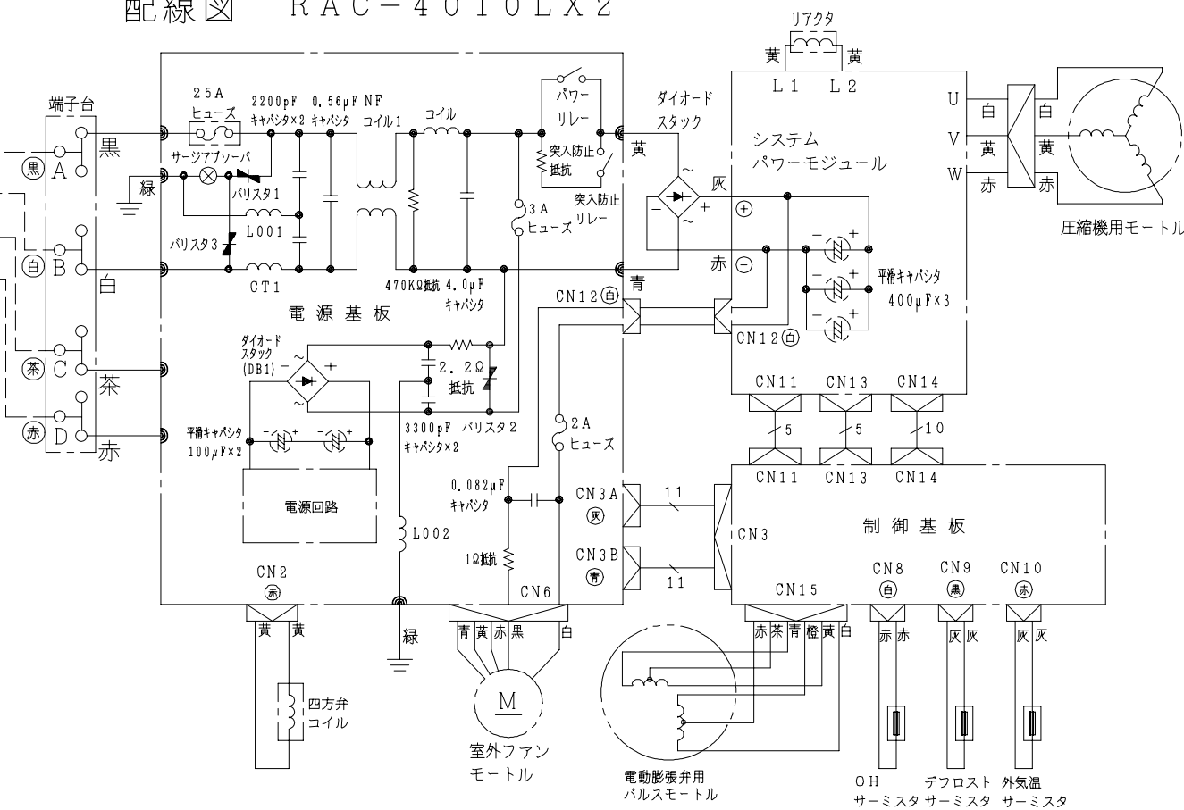
配線図 RAC-4010LX2
