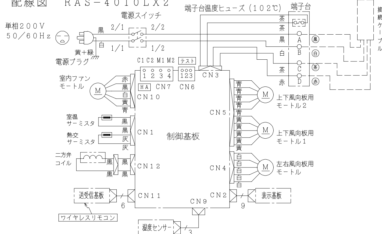
配線図 RAS-4010LX2
